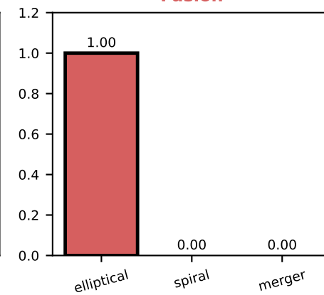
Fusion
