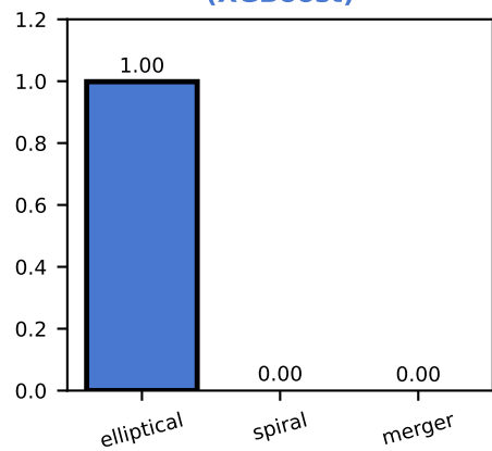
Tabular (XGBoost)
