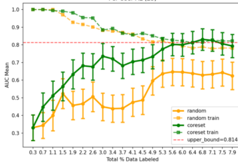
Per-User AL (25)
