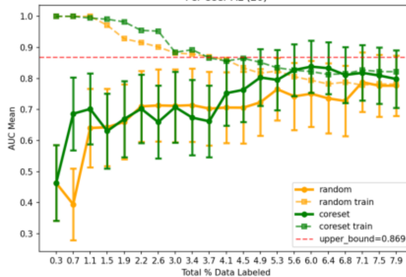
Per-User AL (20)
