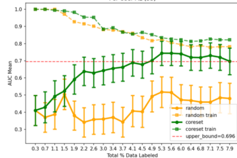
Per-User AL (33)
