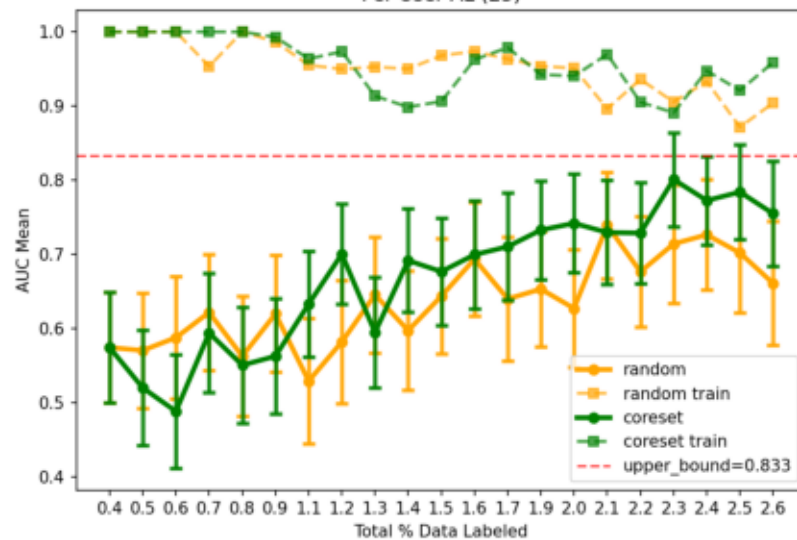
Per-User AL (25)
