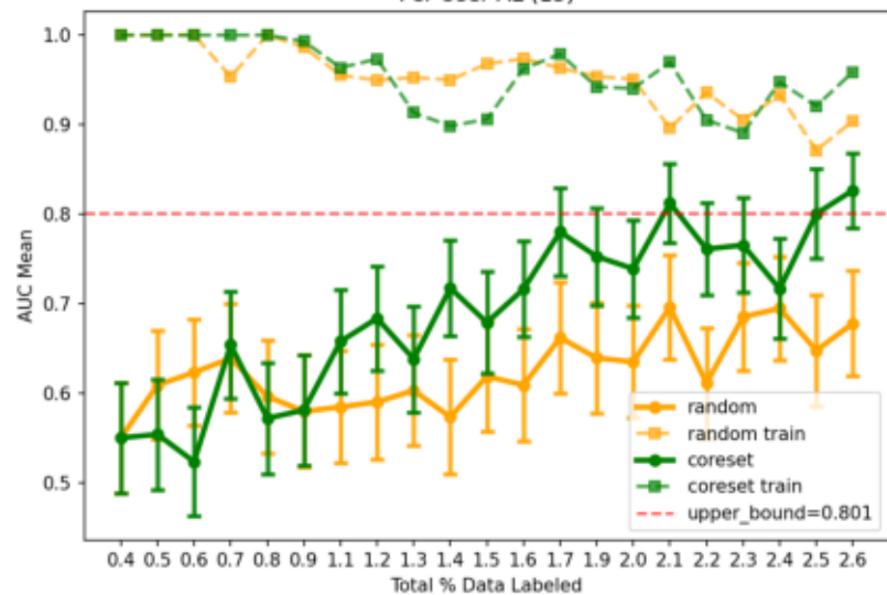
Per-User AL (15)
