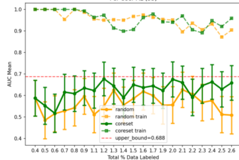
Per-User AL (33)
