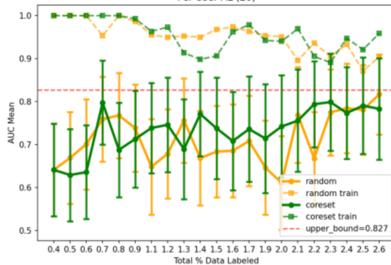
Per-User AL (20)
