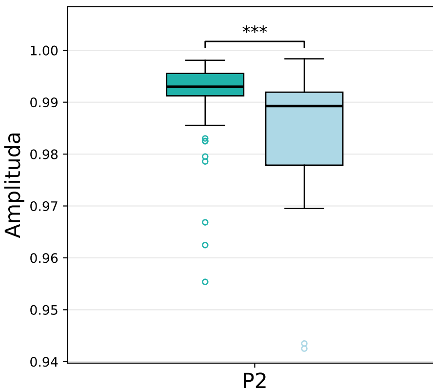
Klasa 4
