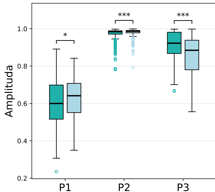
Klasa 3
