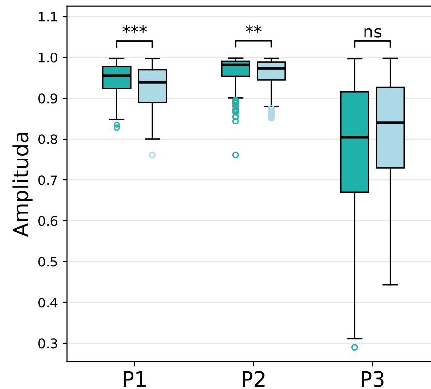
Klasa 2
