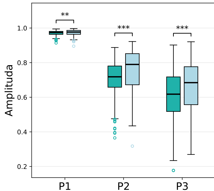
Klasa 1
