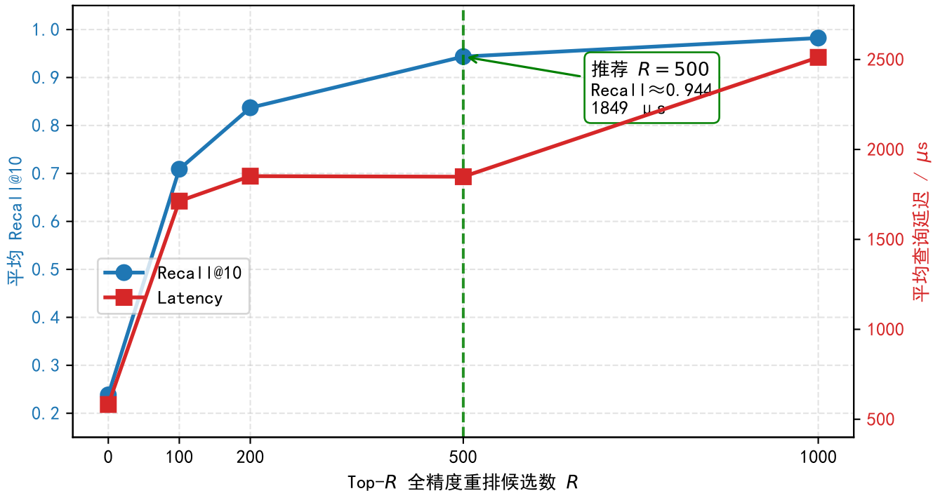
PQ FastScan + Top- R IP 重排: Recall 与延迟随 R 变化 (DEEP100K)
