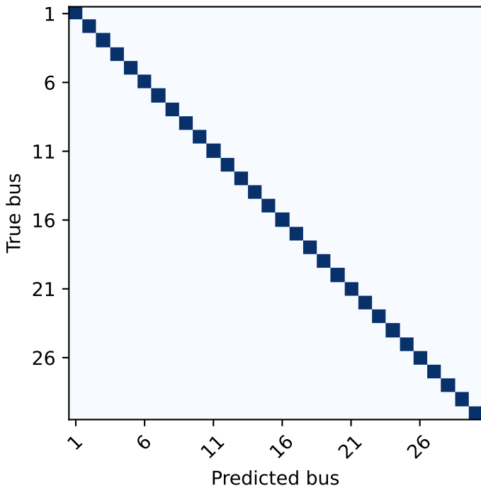
ieee30 Baseline
