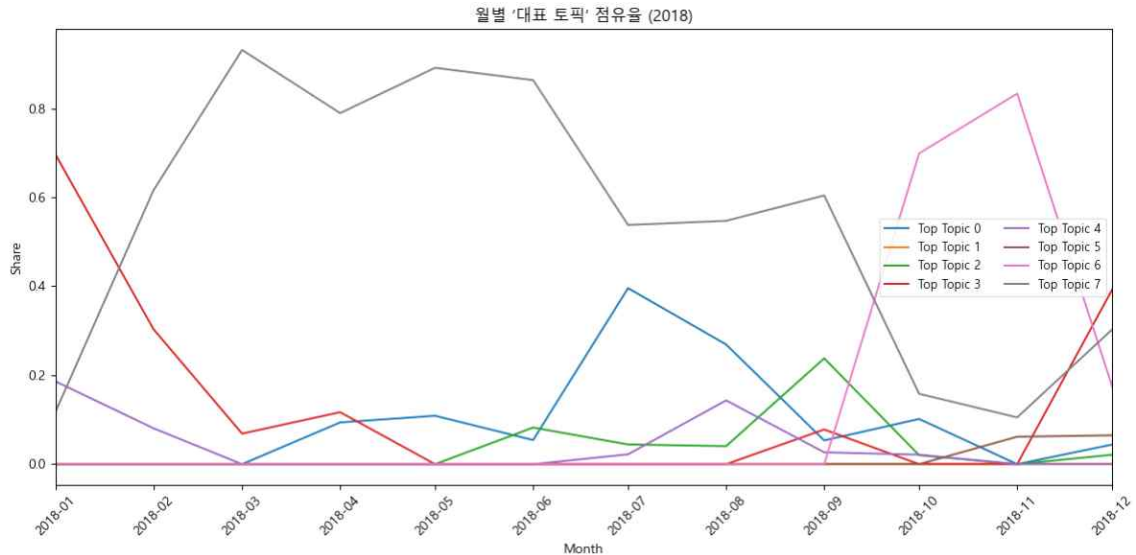
Figure 4. 대표 토픽(문서에서 확률이 가장 높은 토픽)의 점유율
