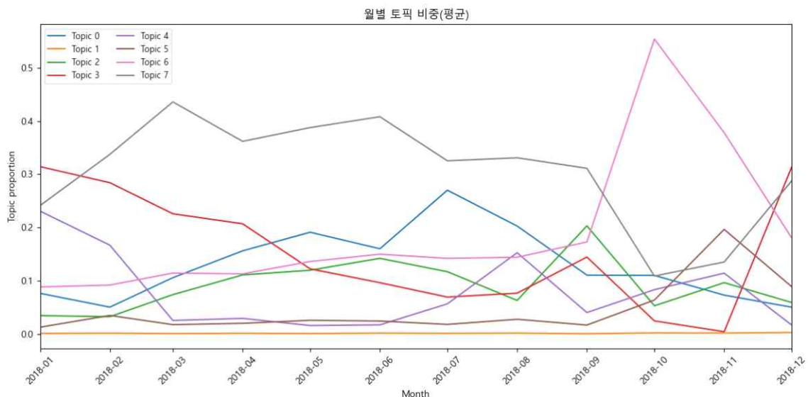
Figure 3. 각 토픽 별 비중의 평균
