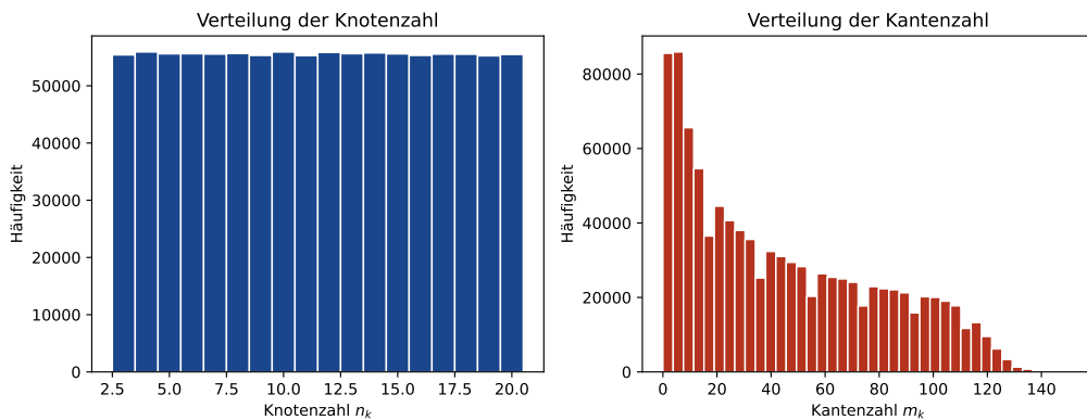
Abbildung 1: Histogramm der Knotenzahl n_k (links, diskret-gleichverteilt auf \{3, \dots, 20\} ) und der Kantenzahl m_k (rechts, approximativ binomialverteilt mit \mathbb{E}[m] \approx p \cdot n(n - 1) ) über alle N = 1.000.000 generierten Netzwerke.
