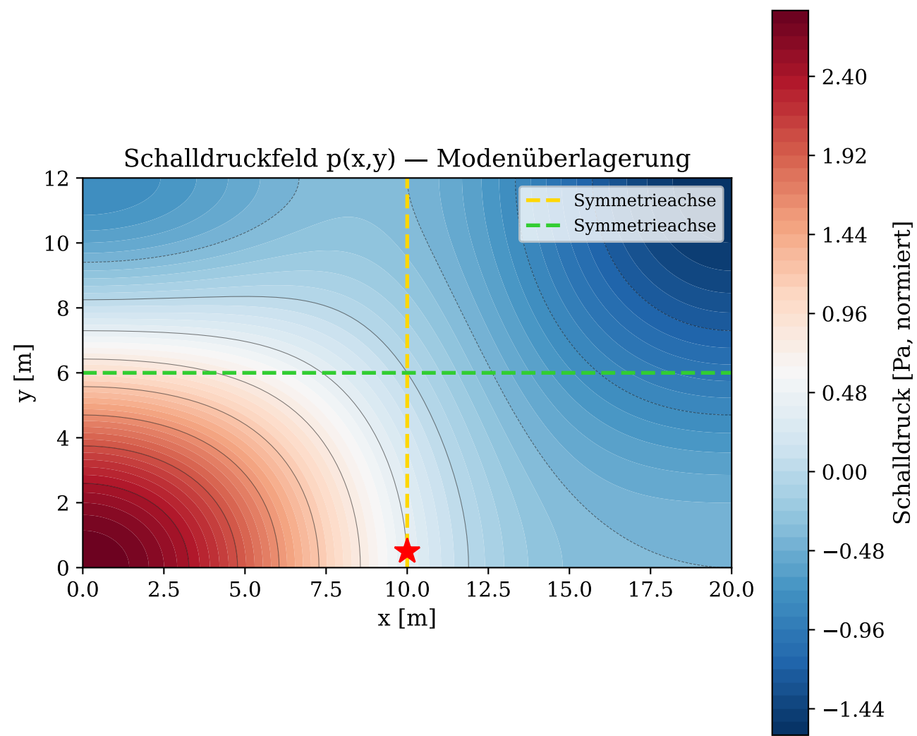
Abbildung 1: Zweidimensionales Schalldruckfeld im symmetrischen Hörsaal
