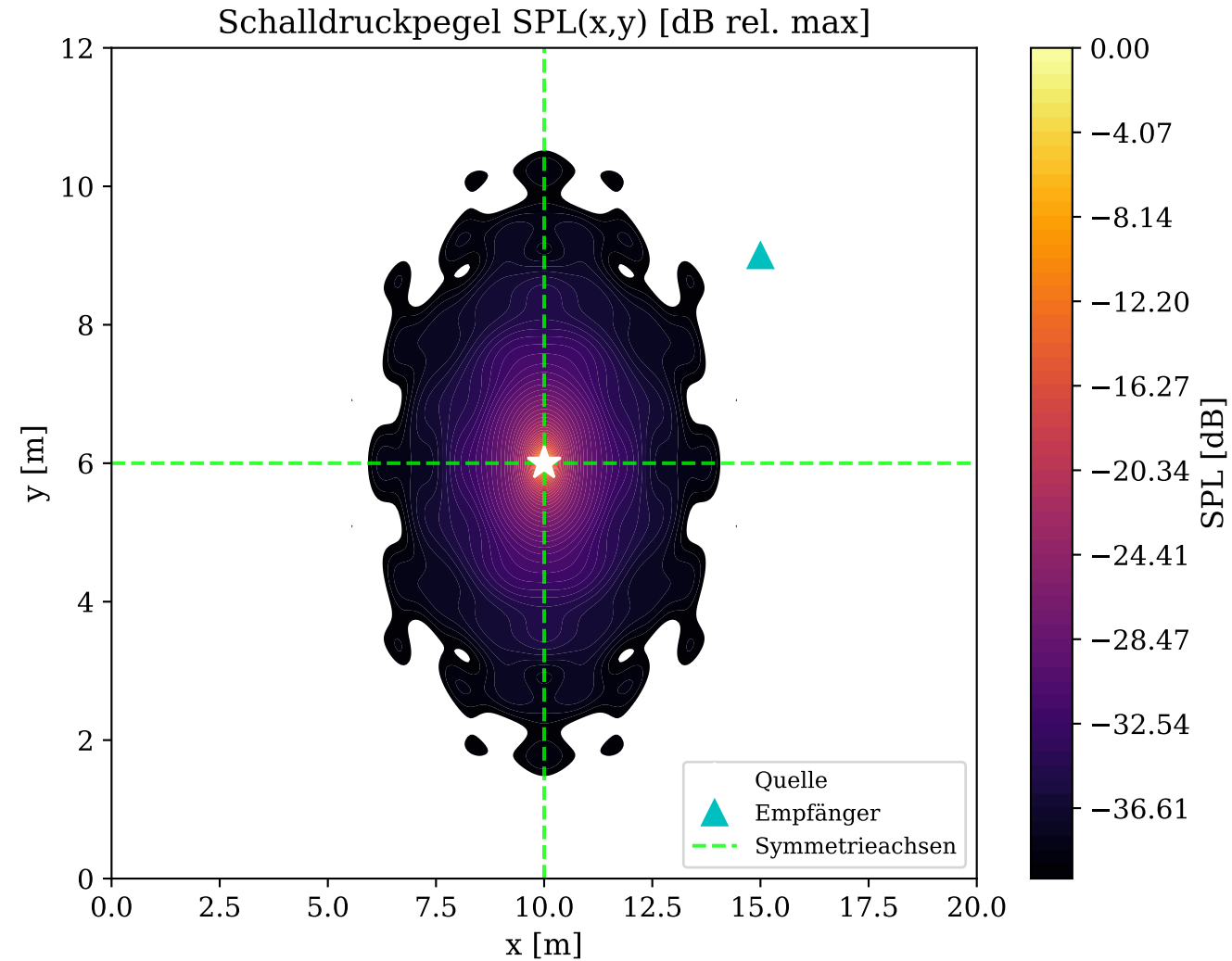
Abbildung 3: Greensche Funktion und Spiegelquellenmethode im symmetrischen Raum
