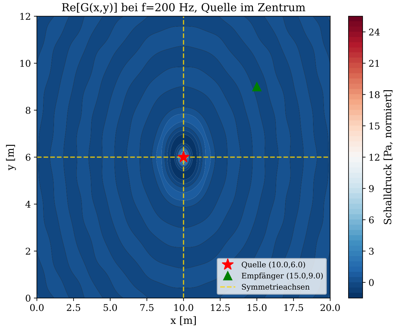
Abbildung 3: Greensche Funktion und Spiegelquellenmethode im symmetrischen Raum
