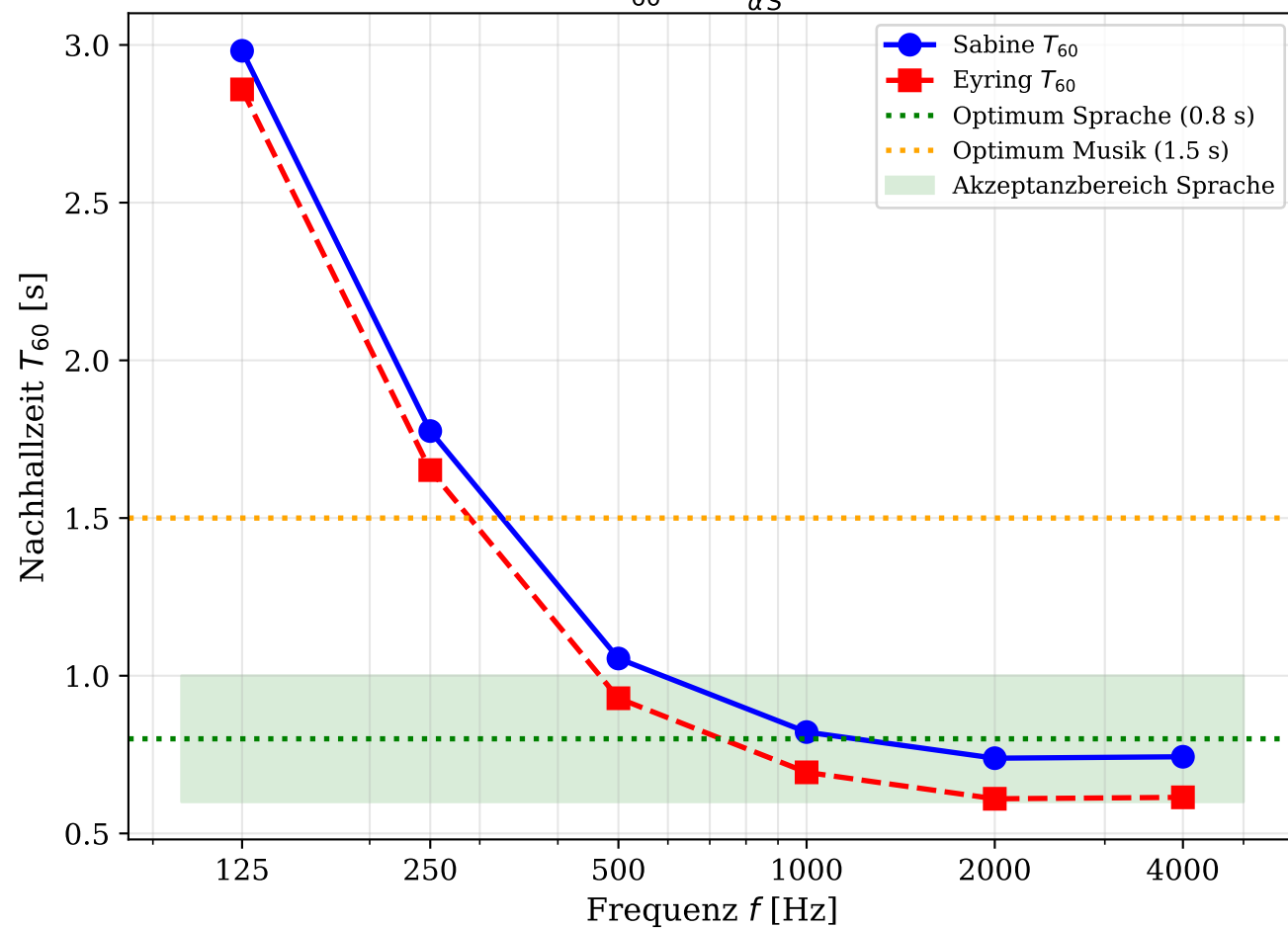
Sabine vs. Eyring Nachhallzeit
