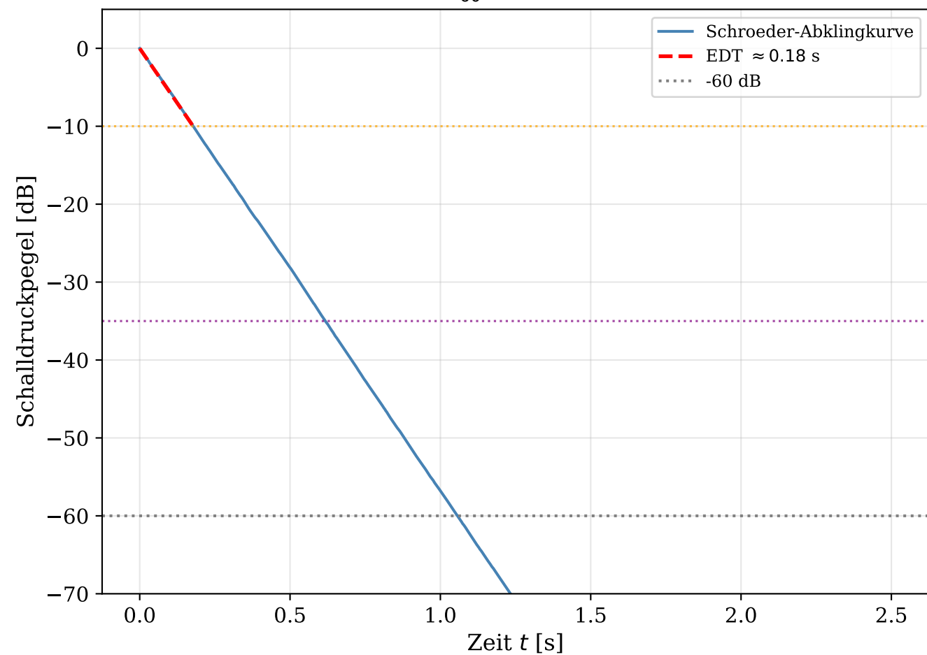
Schroeder-Abklingkurve bei 500 Hz
