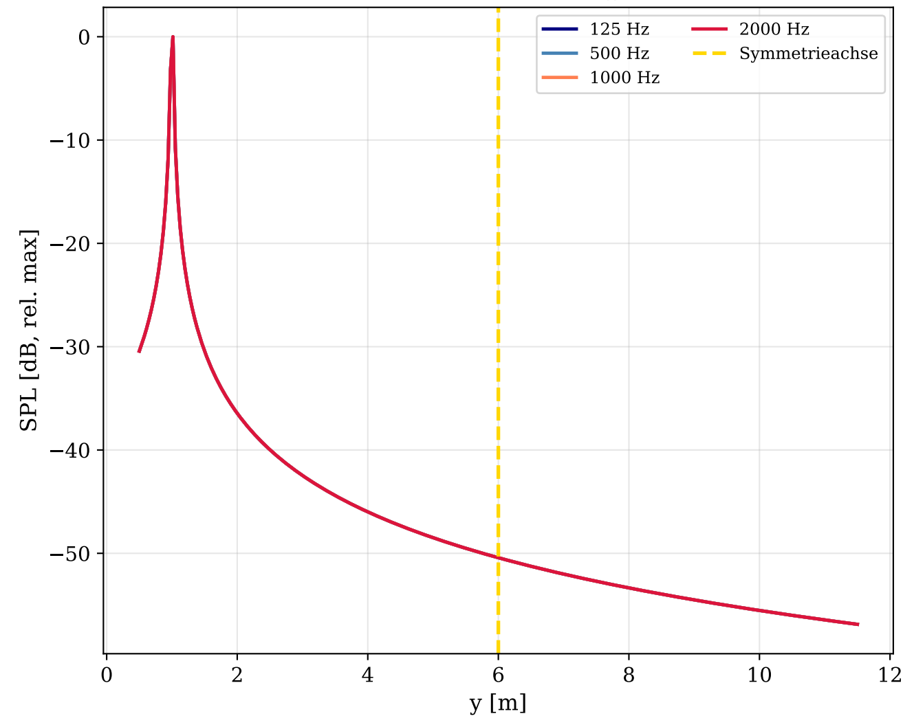
Abbildung 5: Symmetrische Schallpegelverteilung — Profilschnitte und Abweichungsanalyse
