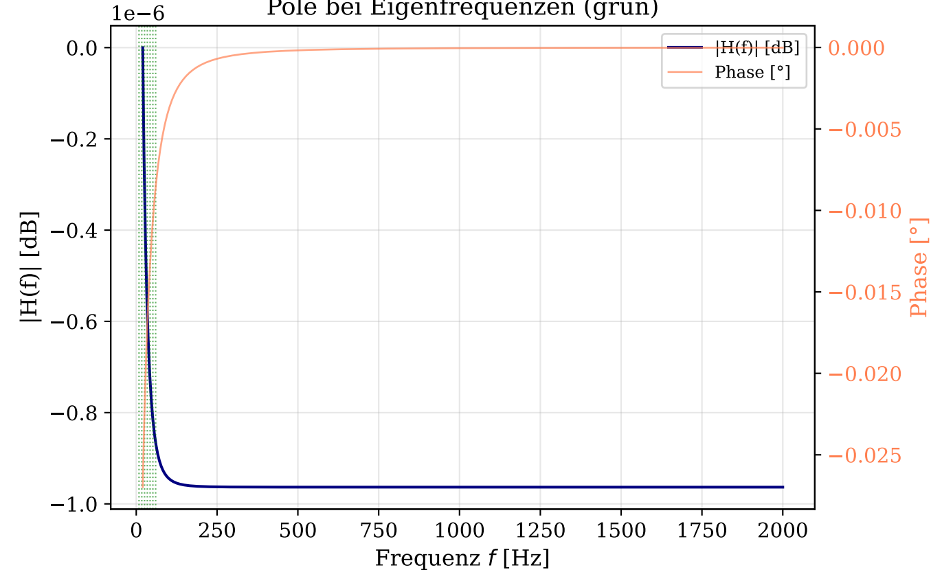
Raumübertragungsfunktion H(f) Pole bei Eigenfrequenzen (grün)
