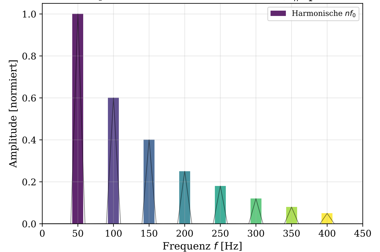
Spektrum: Harmonische Reihe \{nf_0\}_{n=1}^8
