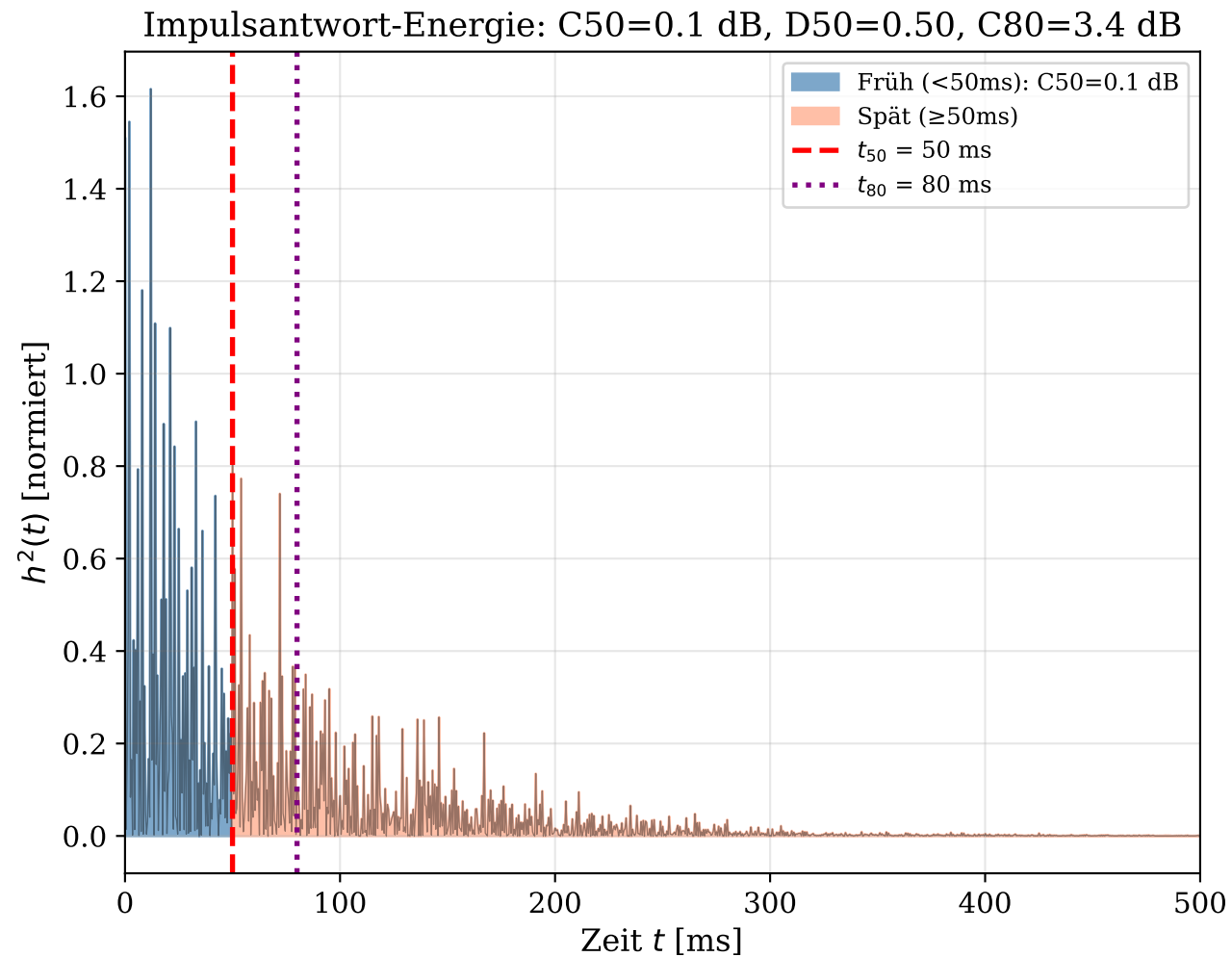
Abbildung 8: Raumakustische Gütekriterien – C50, D50 und Deutlichkeit
