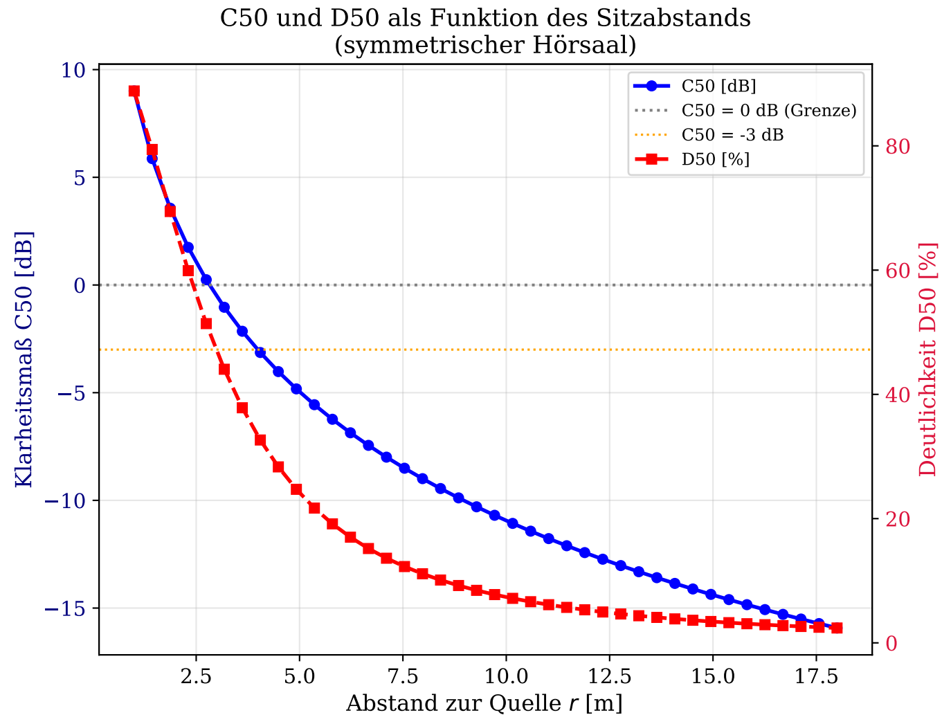
Abbildung 8: Raumakustische Gütekriterien – C50, D50 und Deutlichkeit
