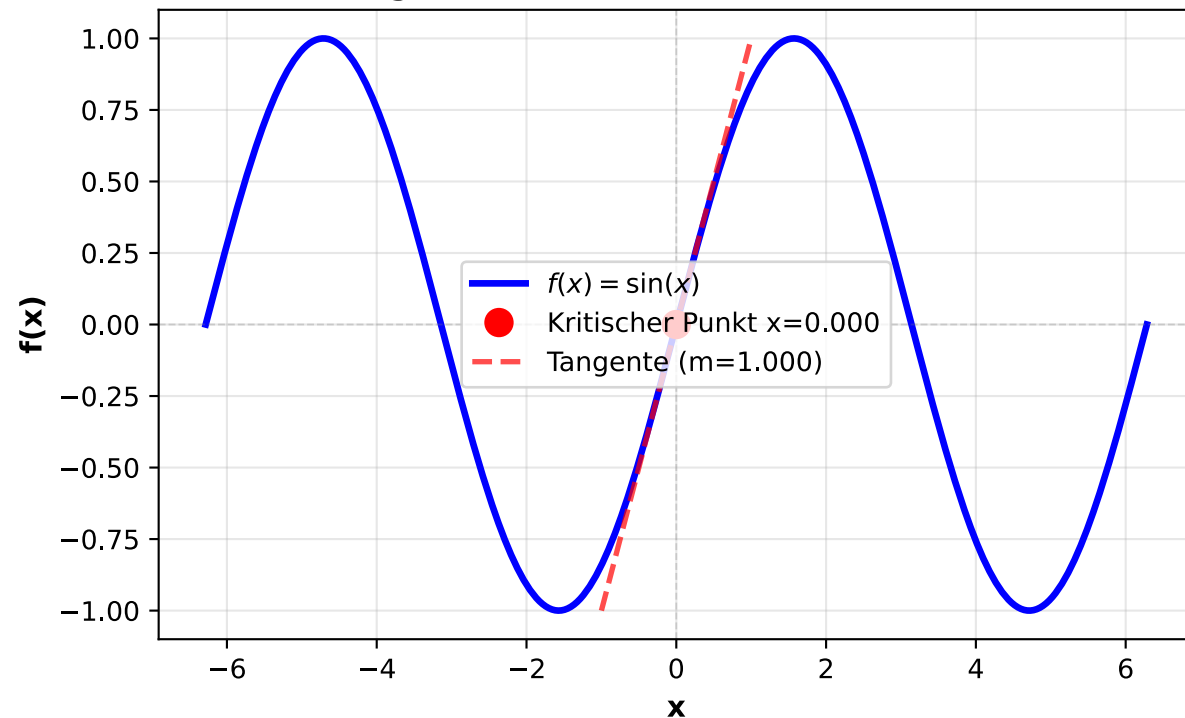
Originalfunktion mit kritischem Punkt
