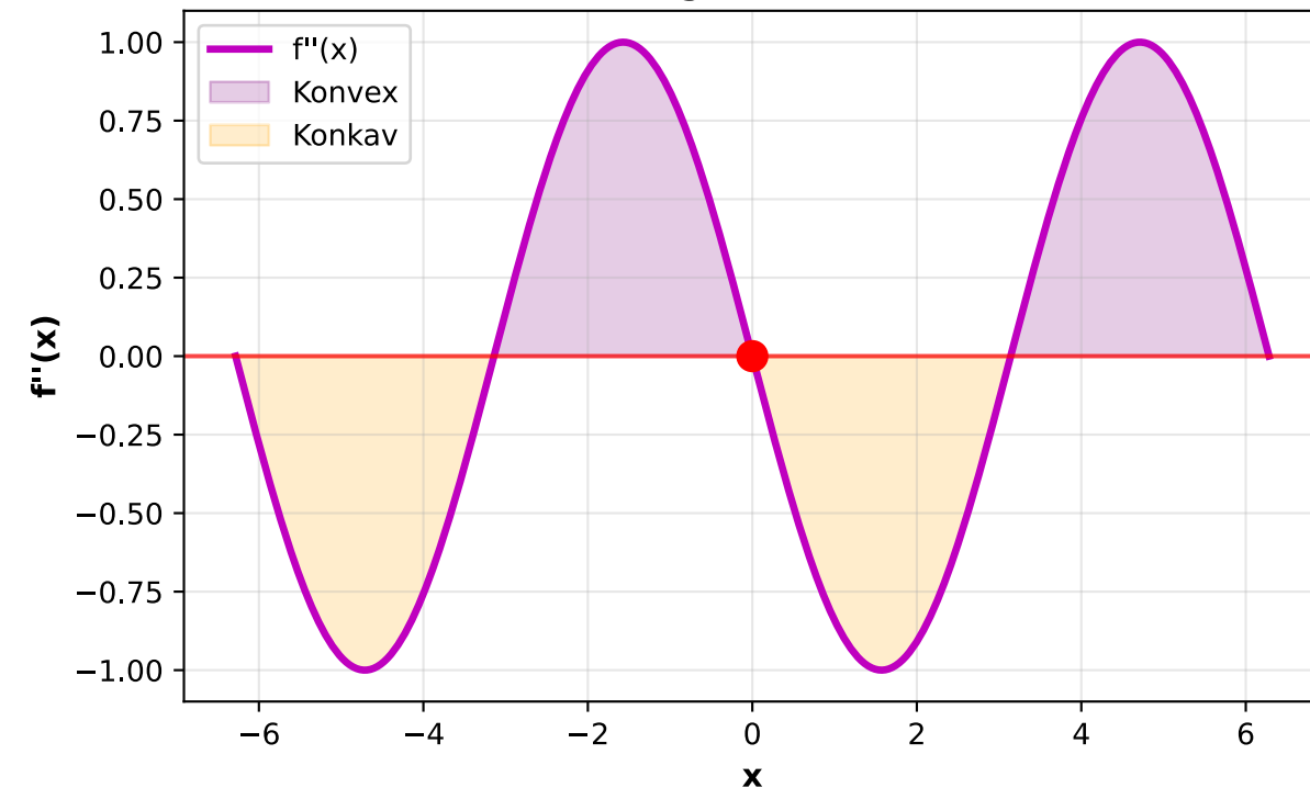
Krümmungsverhalten f''(x)
