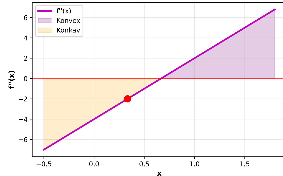
Krümmungsverhalten f''(x)
