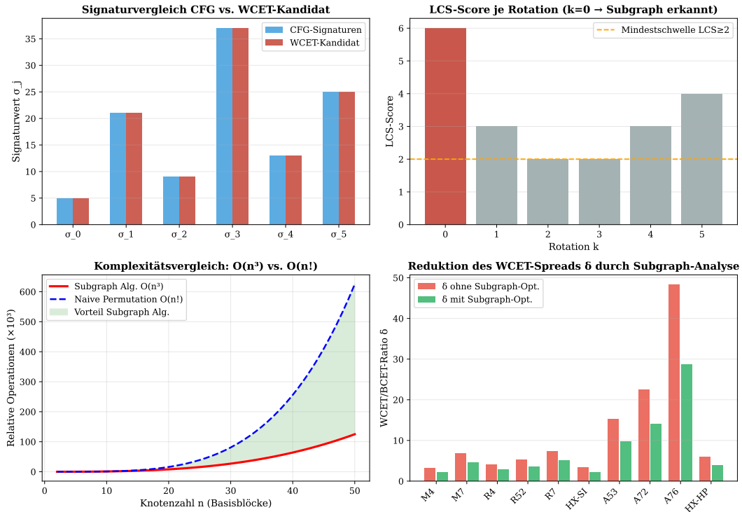
Abbildung W4: Signatur-basierte Zyklusidentifikation im CFG (Subgraph Algorithmus – Rotationsanalyse)
