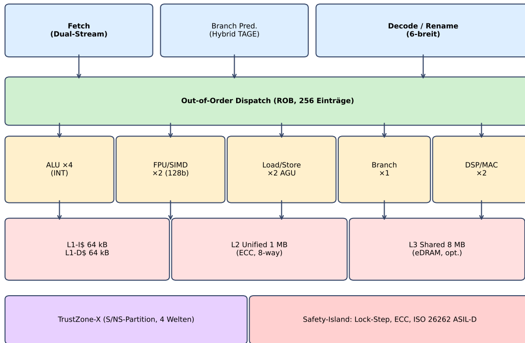
Abbildung 5: Strukturelles Blockdiagramm der Cortex-HX-Architektur (Theorem 6.1).
