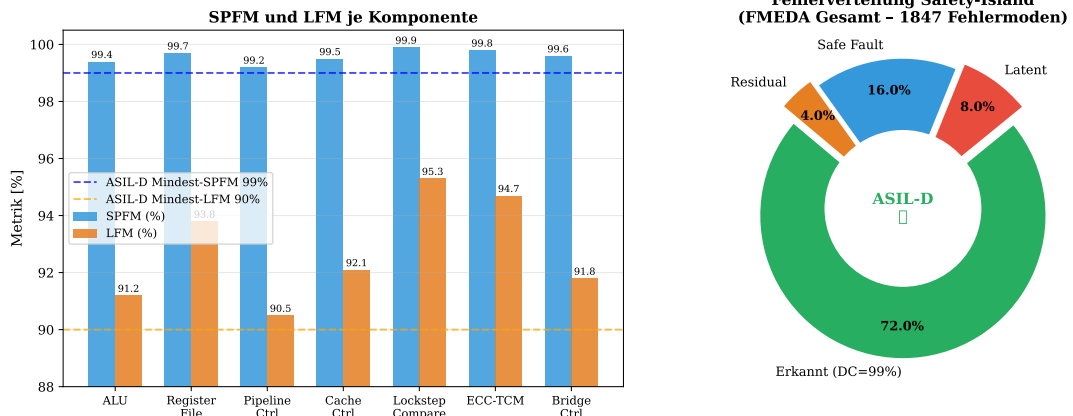
Abbildung R3: FMEDA-Ergebnisse - SPFM und LFM für den Safety-Island (ISO 26262 ASIL-D Nachweis)
