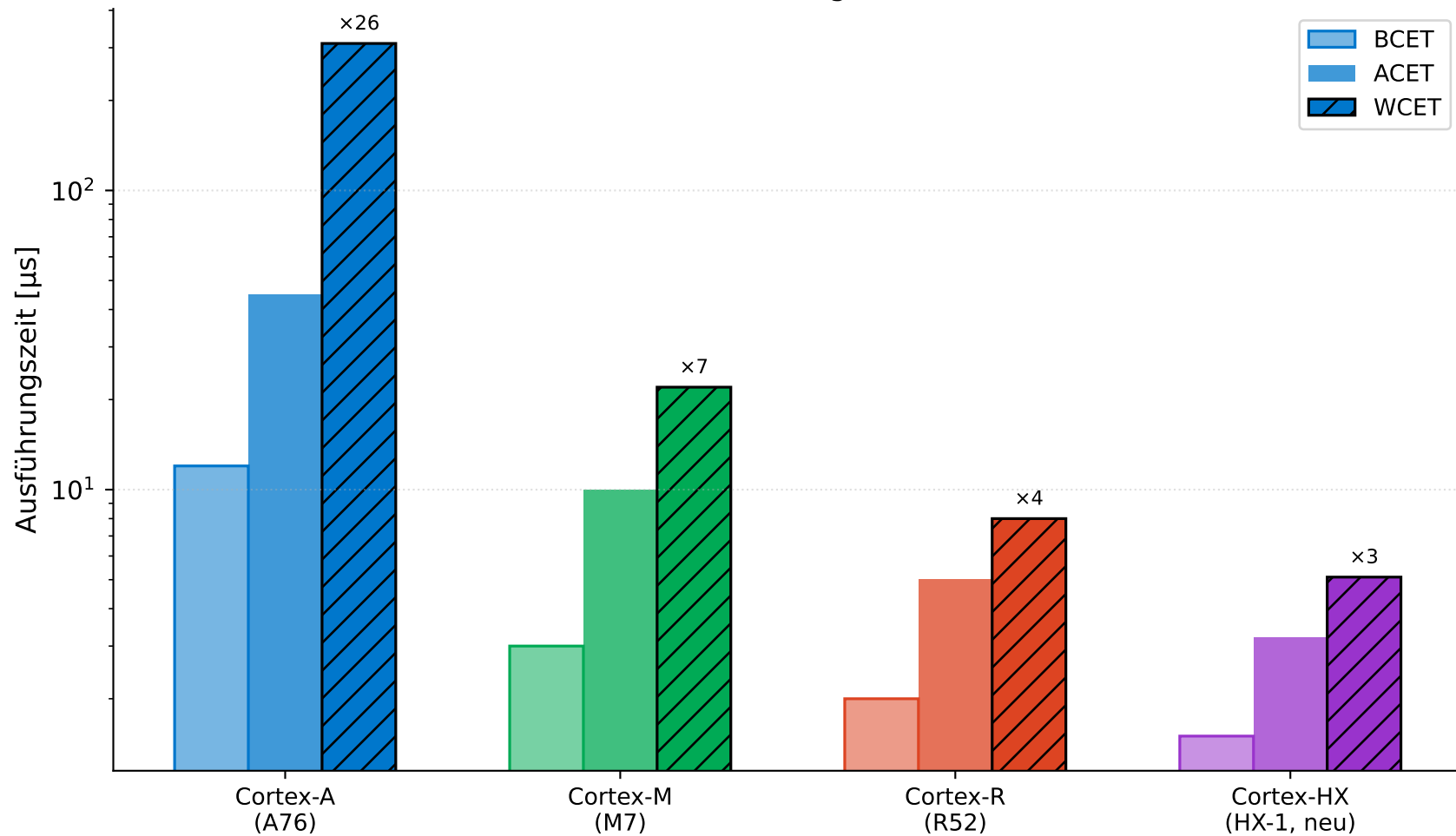
Abb. 2: BCET / ACET / WCET-Vergleich der Cortex-Familien
