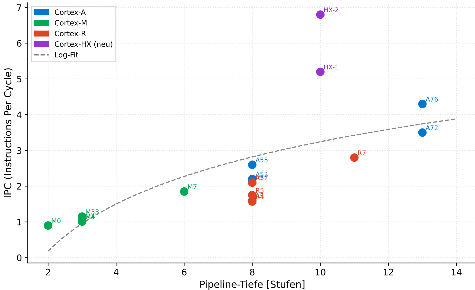
Abb. 3: Pipeline-Tiefe vs. IPC — logarithmisches Skalierungsgesetz
