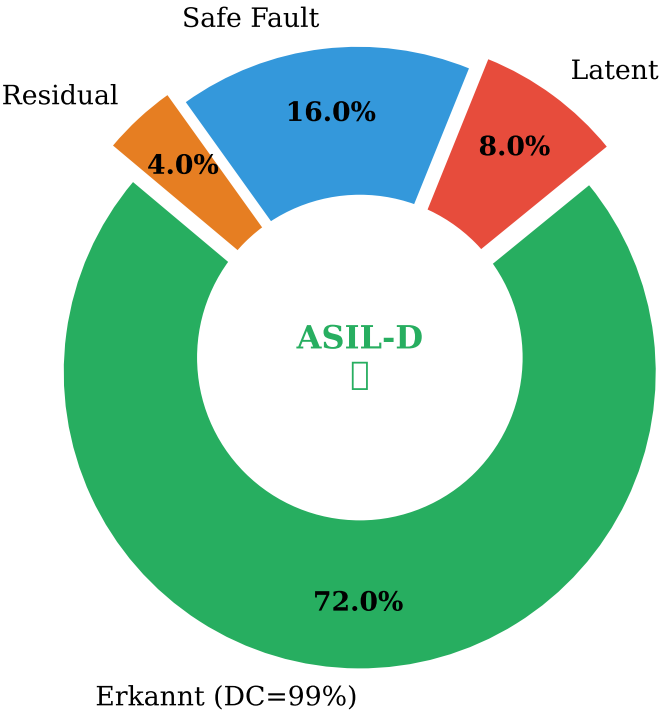
Fehlerverteilung Safety-Island (FMEDA Gesamt - 1847 Fehlermoden)
