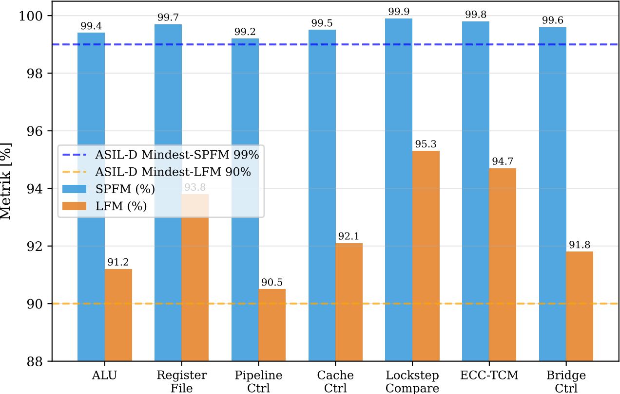
SPFM und LFM je Komponente
