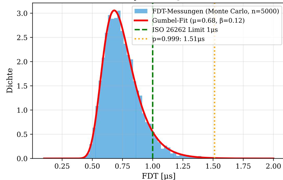
FDT-Verteilung (Monte Carlo Simulation) Safety-Island @2GHz
