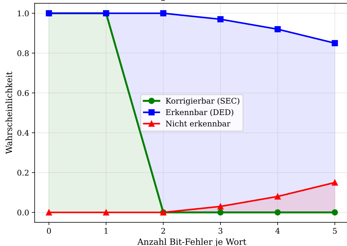
SECDED-Fähigkeit vs. Bit-Fehleranzahl
