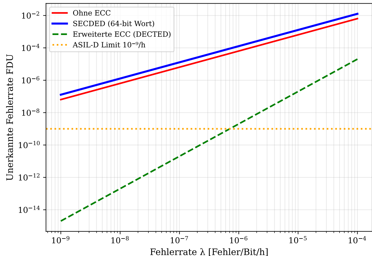
Unerkannte Fehlerrate FDU vs. Einzel-Fehlerrate \lambda
