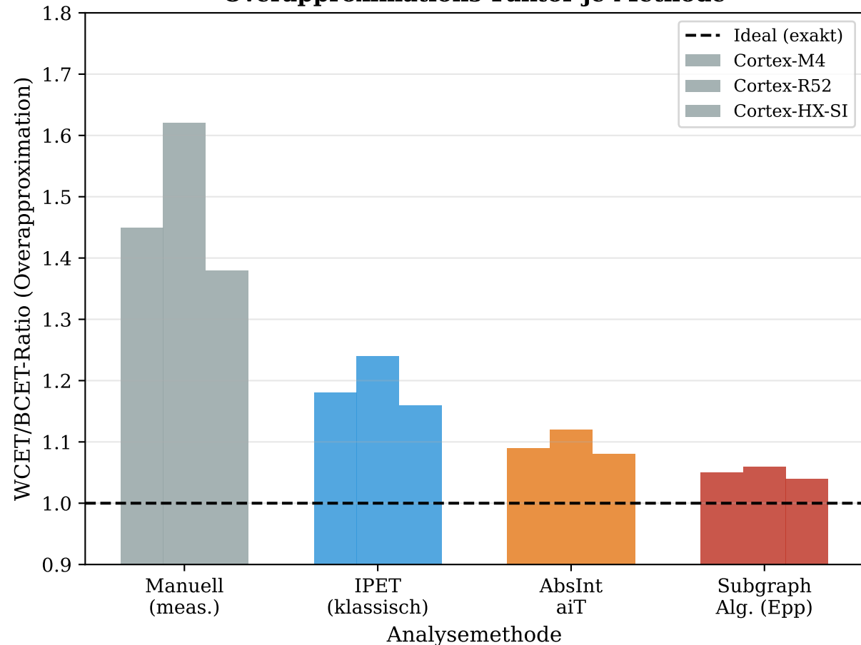
Overapproximations-Faktor je Methode
