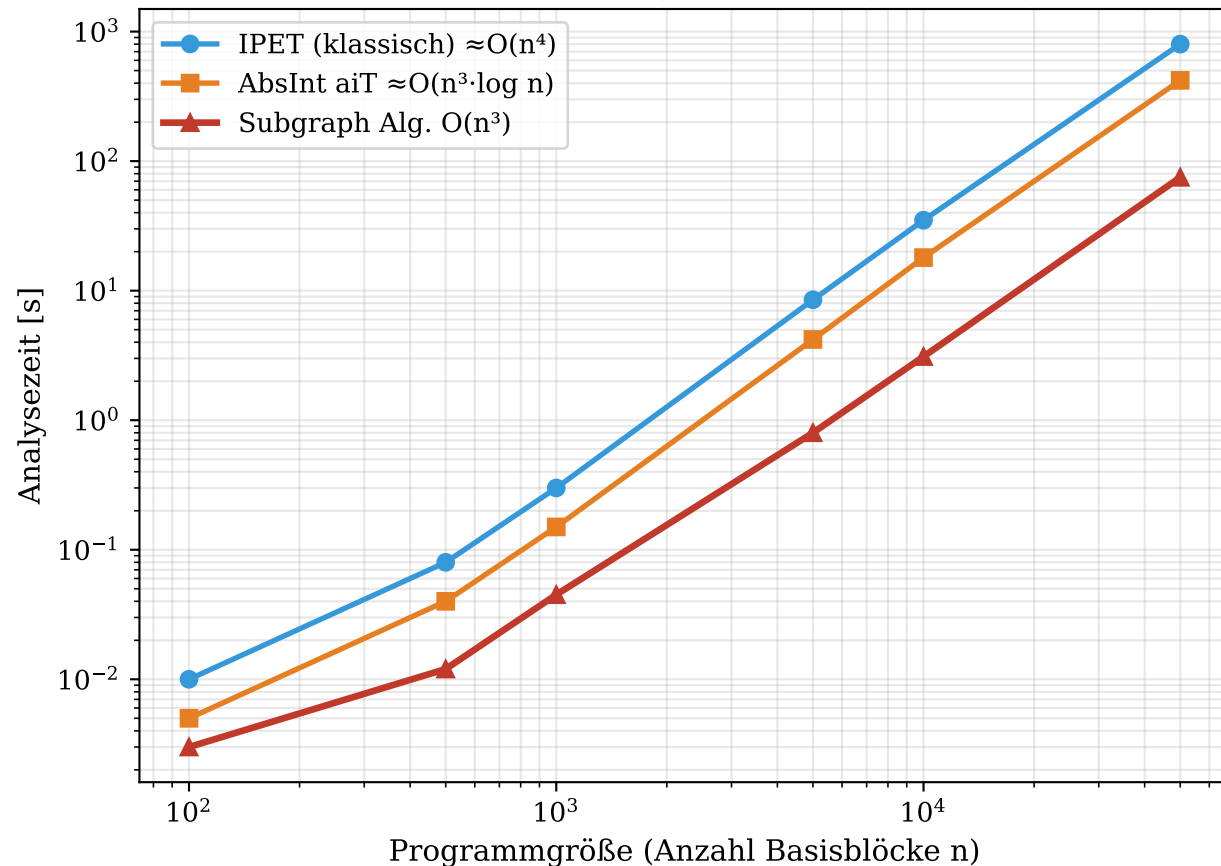
Laufzeit-Skalierung O(n^3) Subgraph Alg.
