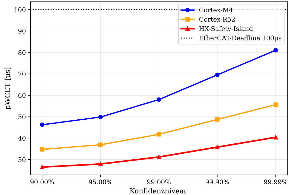
pWCET vs. Konfidenzniveau (EtherCAT-Deadline 100 \mu\text{s} )
