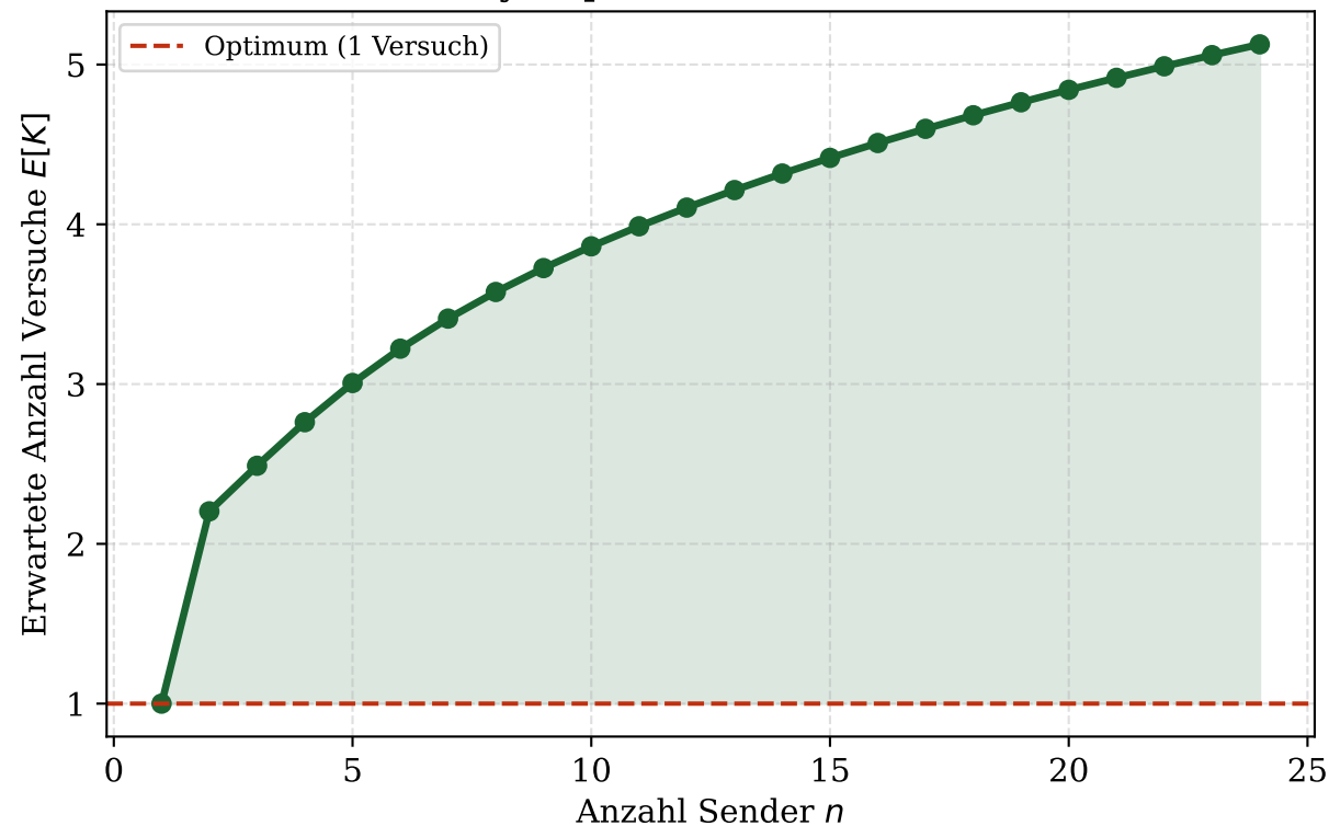
Erwartete Versuche bis Erfolg (Binary Exp. Backoff, IEEE 802.3)
