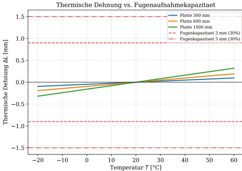
Abbildung 2: Thermische Dehnung dreier Plattenformate im Vergleich zur Fugenaufnahmekapazität bei w = 3 mm (gestrichelt) und w = 5 mm (strichpunktirt).
