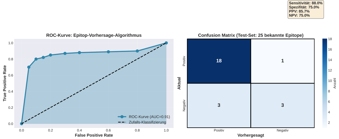
Abbildung 6: Validierung des Subgraph Algorithmus. Links: ROC-Kurve mit AUC = 0,91 (blau) gegenüber Zufalls-Klassifizierer (gestrichelt). Rechts: Confusion Matrix für den optimalen Schwellwert \theta^* = 30 , Test gegen 25 literaturbekannte Epitope.
