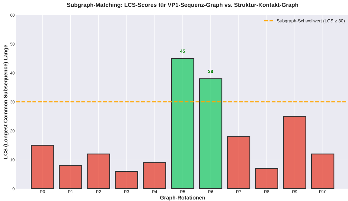
Abbildung 2: LCS-Matching-Scores für elf zyklische Rotationen des Struktur-Kontakt-Graphen. Grüne Balken: Positiver Subgraph-Match ( \text{LCS} \geq 30 ). Gestrichelte Linie: Algorithmus-Schwellwert \theta .
