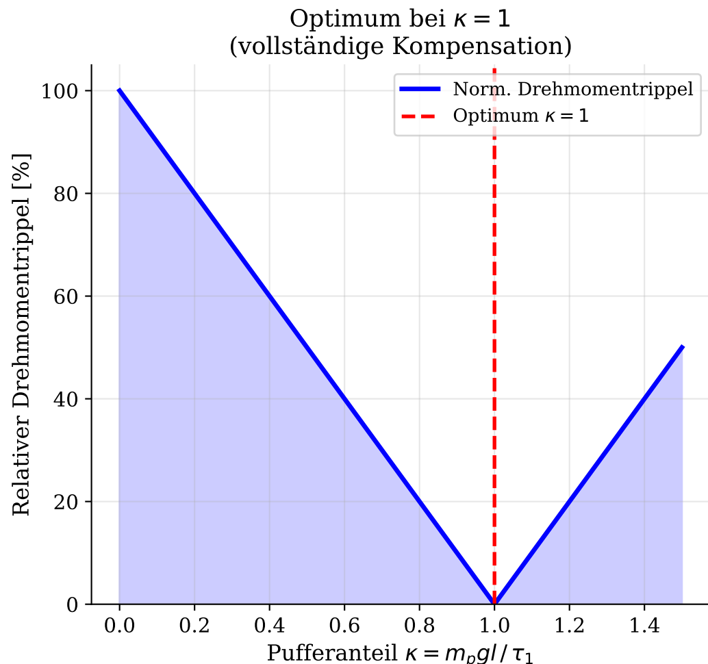
Abbildung 10 - Synergiekonzepte I & II: Gravitation + Elektromotor
