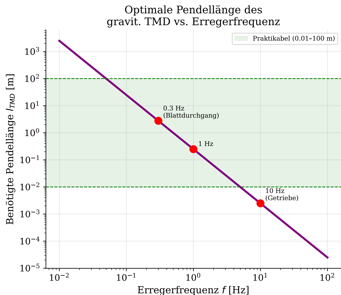
Abbildung 12 - Gravitativer TMD und Magnetmaterial-Vergleich
