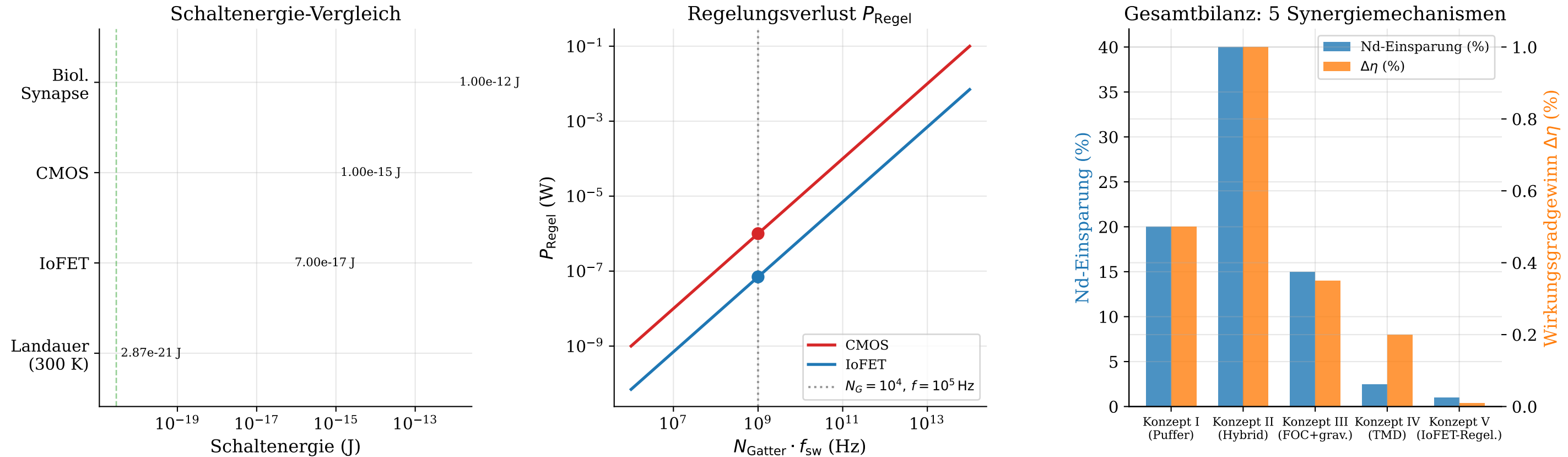
Abbildung 16 - IoFET-Regelungselektronik in der PMSM-Verlustbilanz
