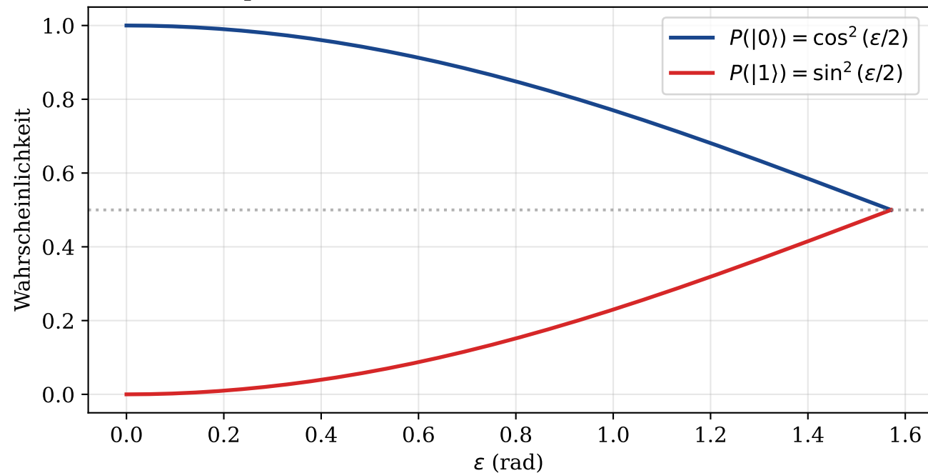
Einzelqubit-Messwahrscheinlichkeit vs. Phasenfehler \varepsilon
