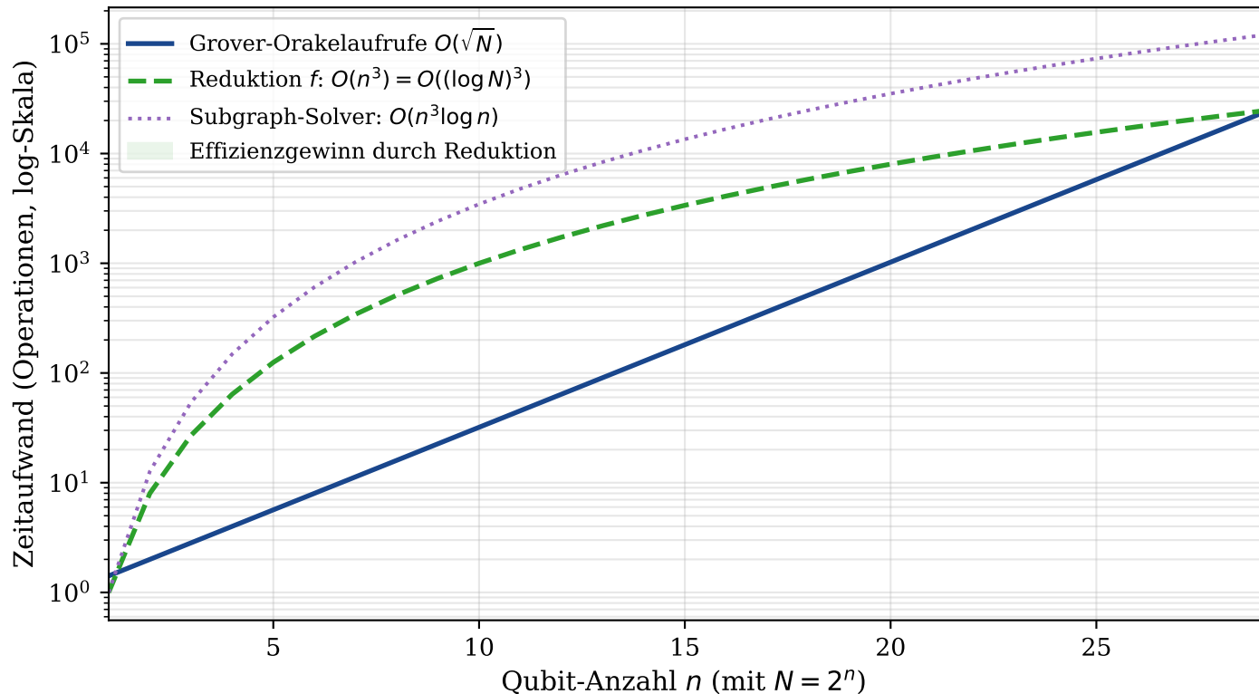
Plot 5 — Laufzeitkosten der Reduktionsfunktion f vs. Grover
