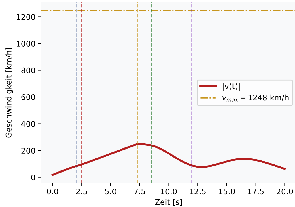
Geschwindigkeitsprofil v(t)
