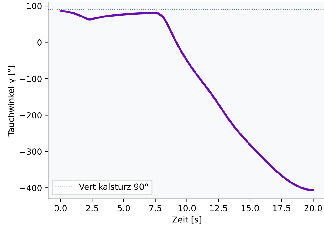
Tauchwinkel \gamma(t)
