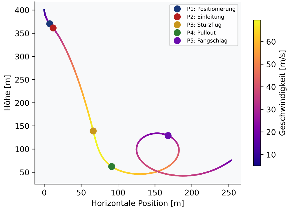
Sturzflugtrajektorie (farbkodiert nach v)
