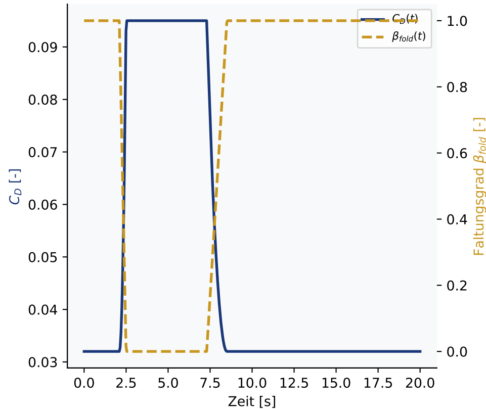
Widerstandsbeiwert & Flügelfalte
