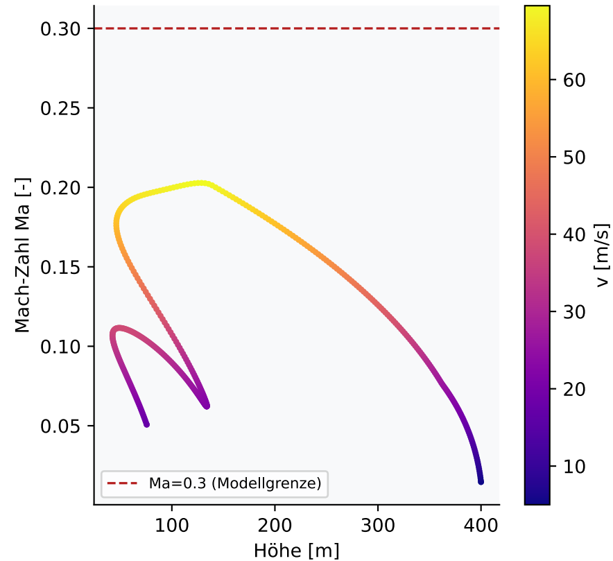
Mach-Zahl über Höhe
