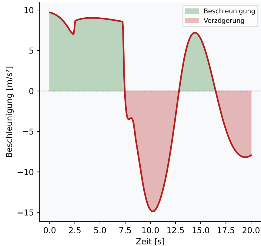
Beschleunigungsprofil a(t)
