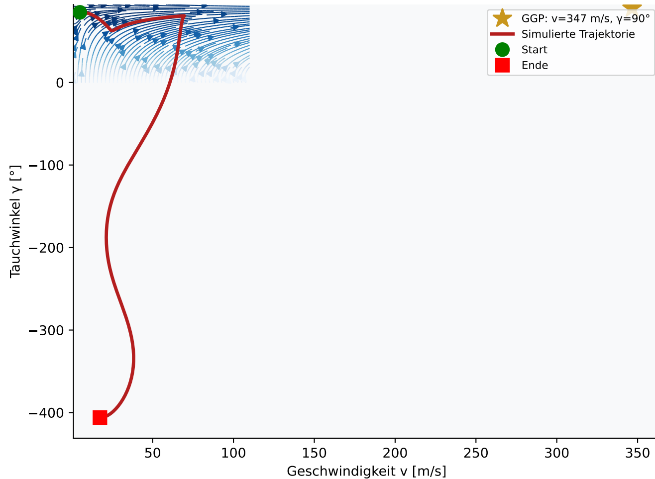
(v, \gamma) -Phasenraum
