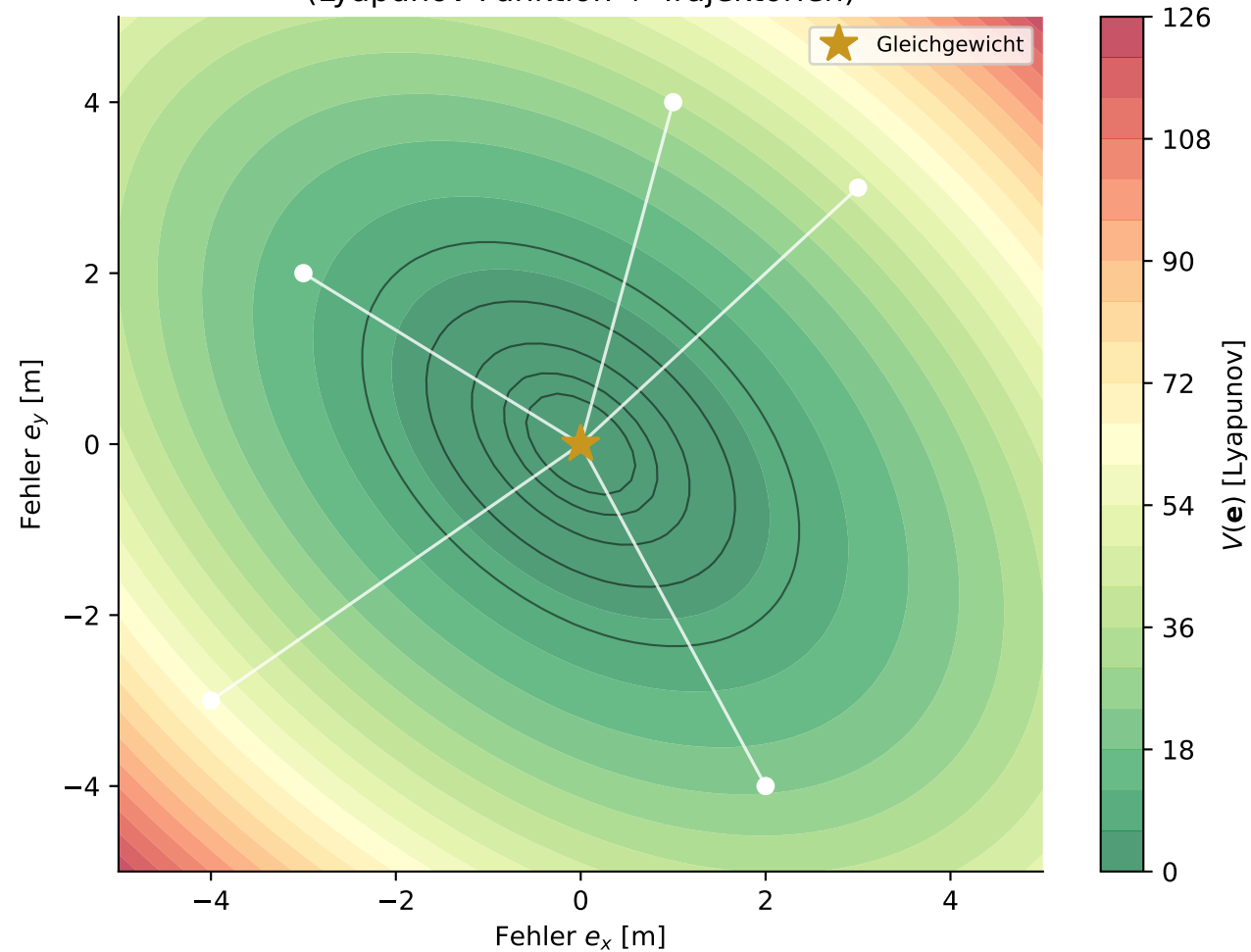
Attraktorbecken des BGS-G-Reglers (Lyapunov-Funktion + Trajektorien)
