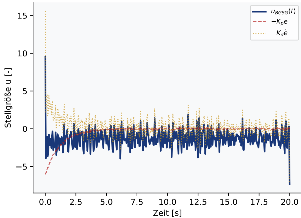
Stellgrößen u(t)
