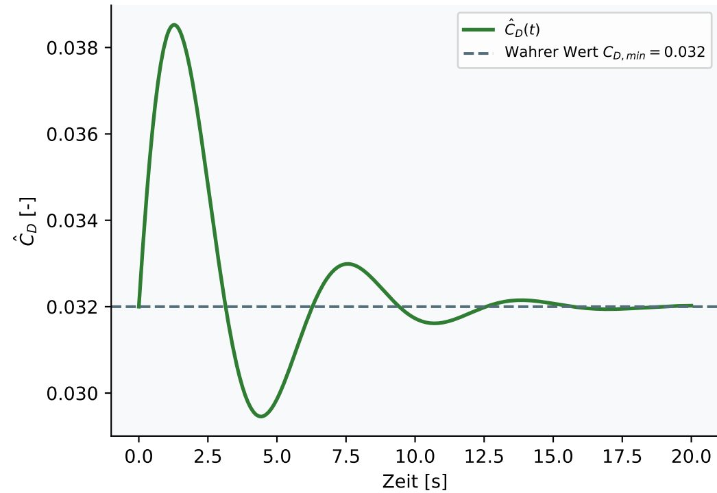
Adaptiver Parameter \hat{C}_D(t)
