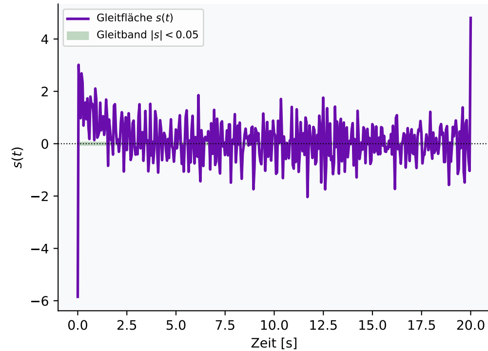
Gleitflächenvariable s(t) = \dot{e} + \Lambda e
