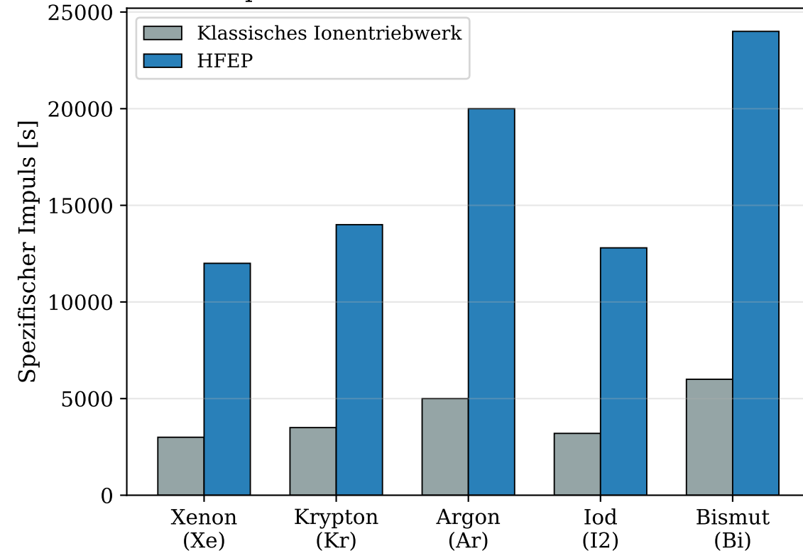
Isp nach Treibstoff: Klassisch vs. HFEP
