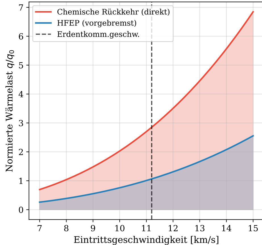
Wiedereintrittserwärmung
