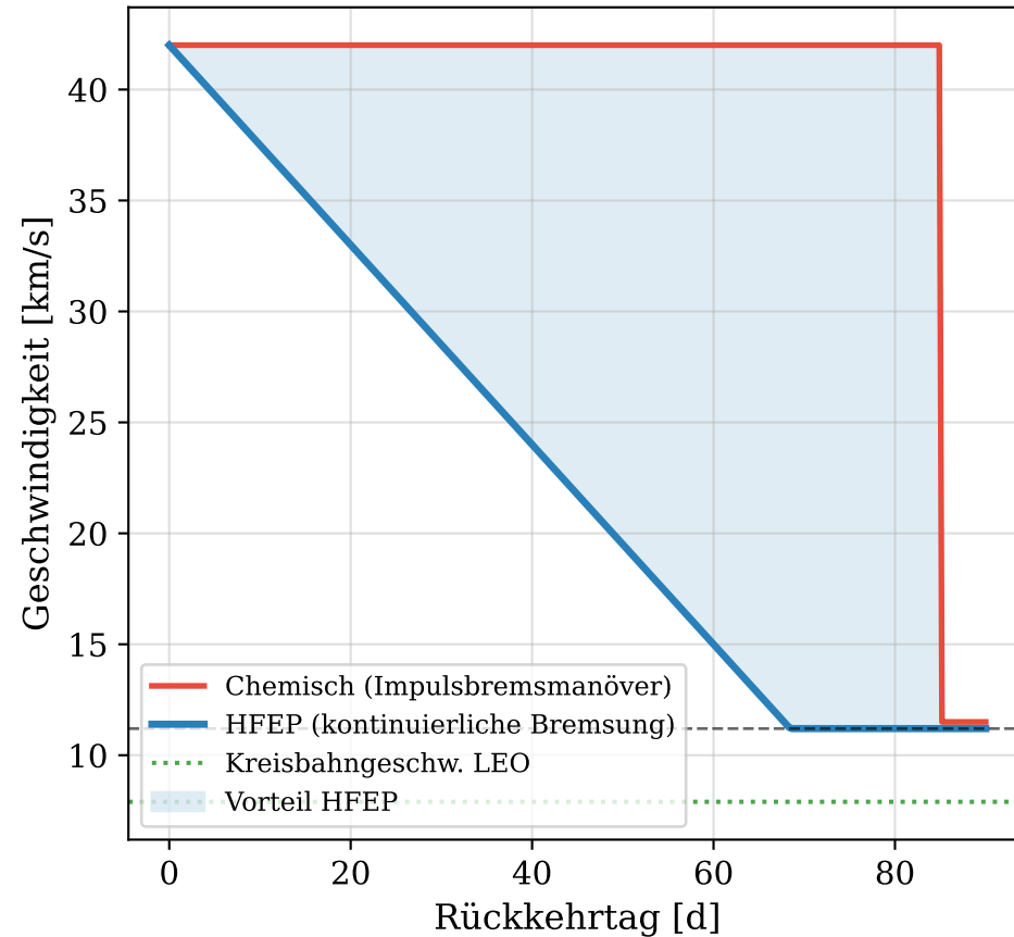
Rückkehrbremsung: Strategie
