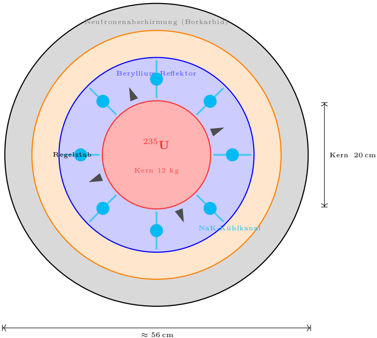
KSR-2 Reaktorquerschnitt
