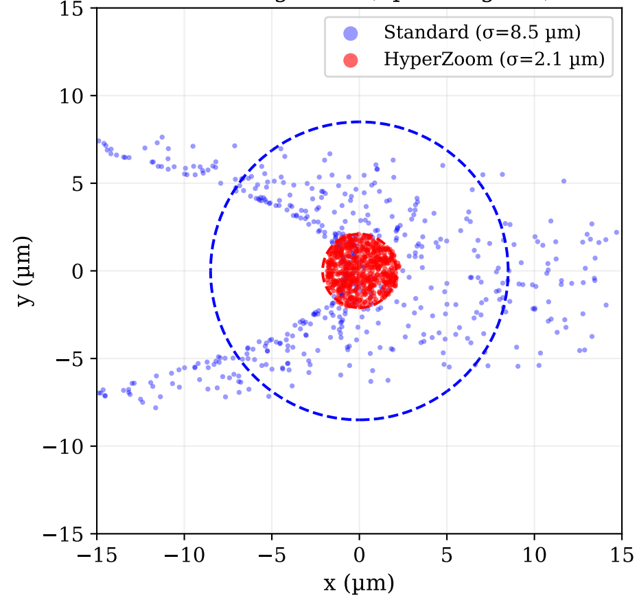
Punkttdiagramm (Spot Diagram)
