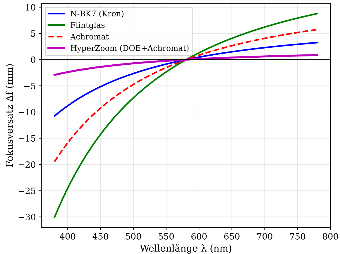
Chromatische Aberration und Korrektur
