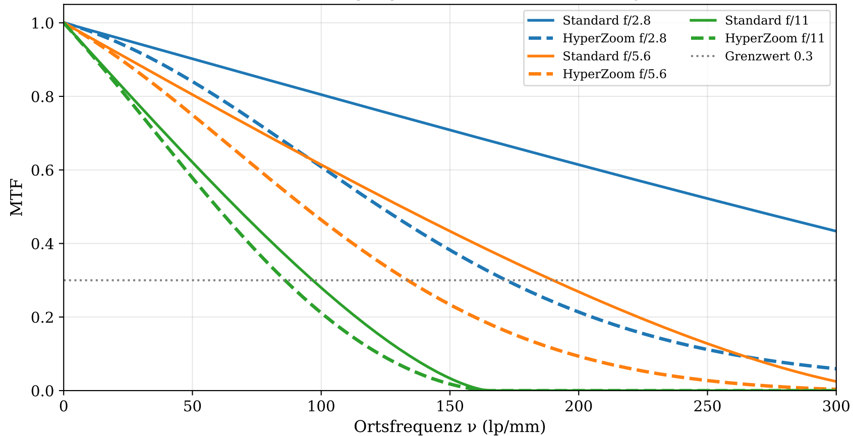
Modulationsübertragungsfunktion – Standard vs. HyperZoom
