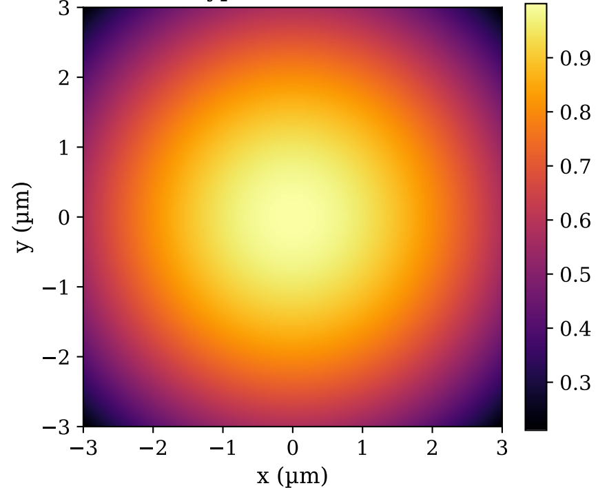
PSF HyperZoom (schärfer)
