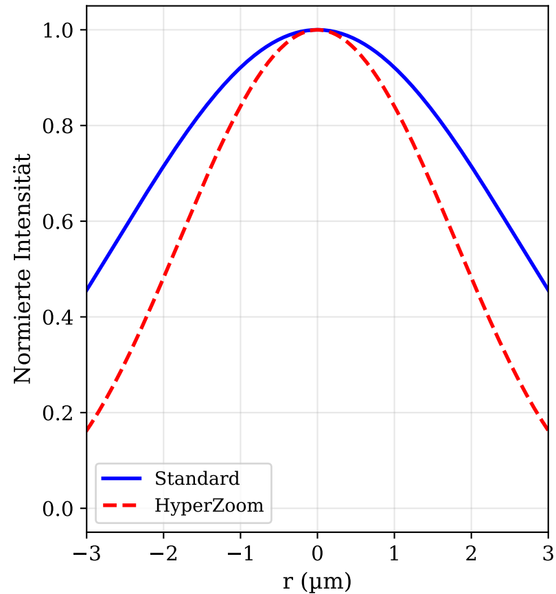
PSF – radialer Schnitt
