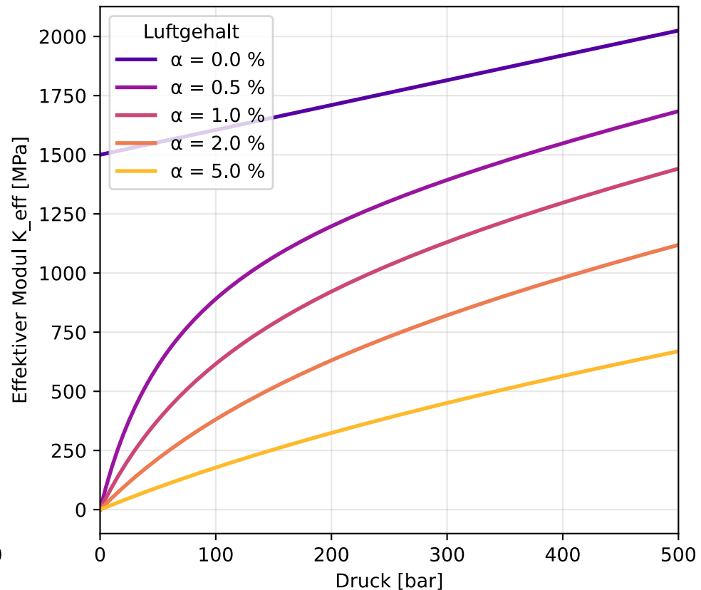
Effektiver Modul mit entlüftetem Anteil \alpha
