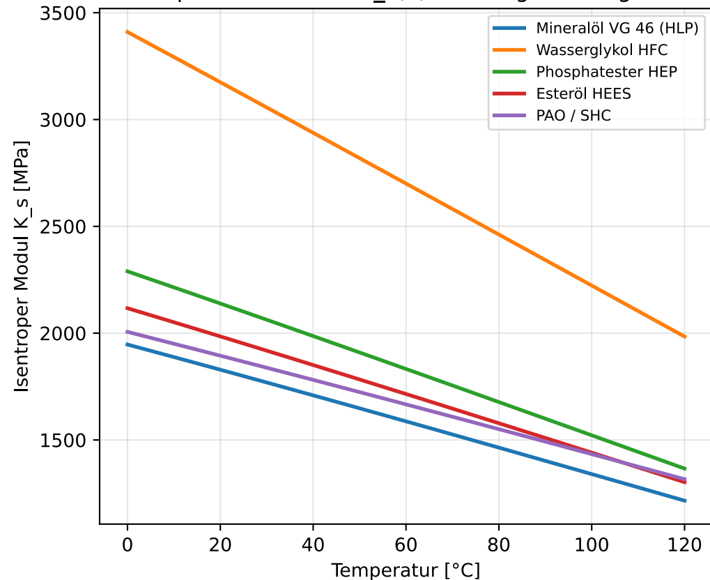
Kompressionsmodul K_s(T) – Flüssigkeitsvergleich
