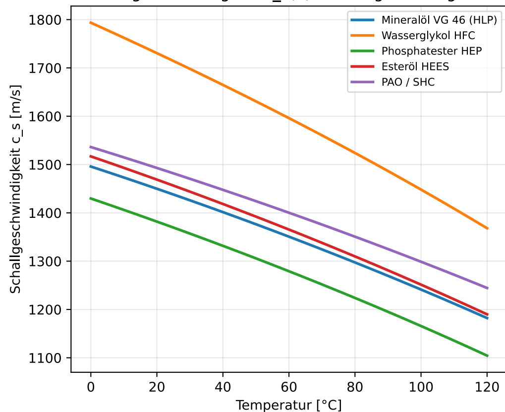
Schallgeschwindigkeit c_s(T) – Flüssigkeitsvergleich
