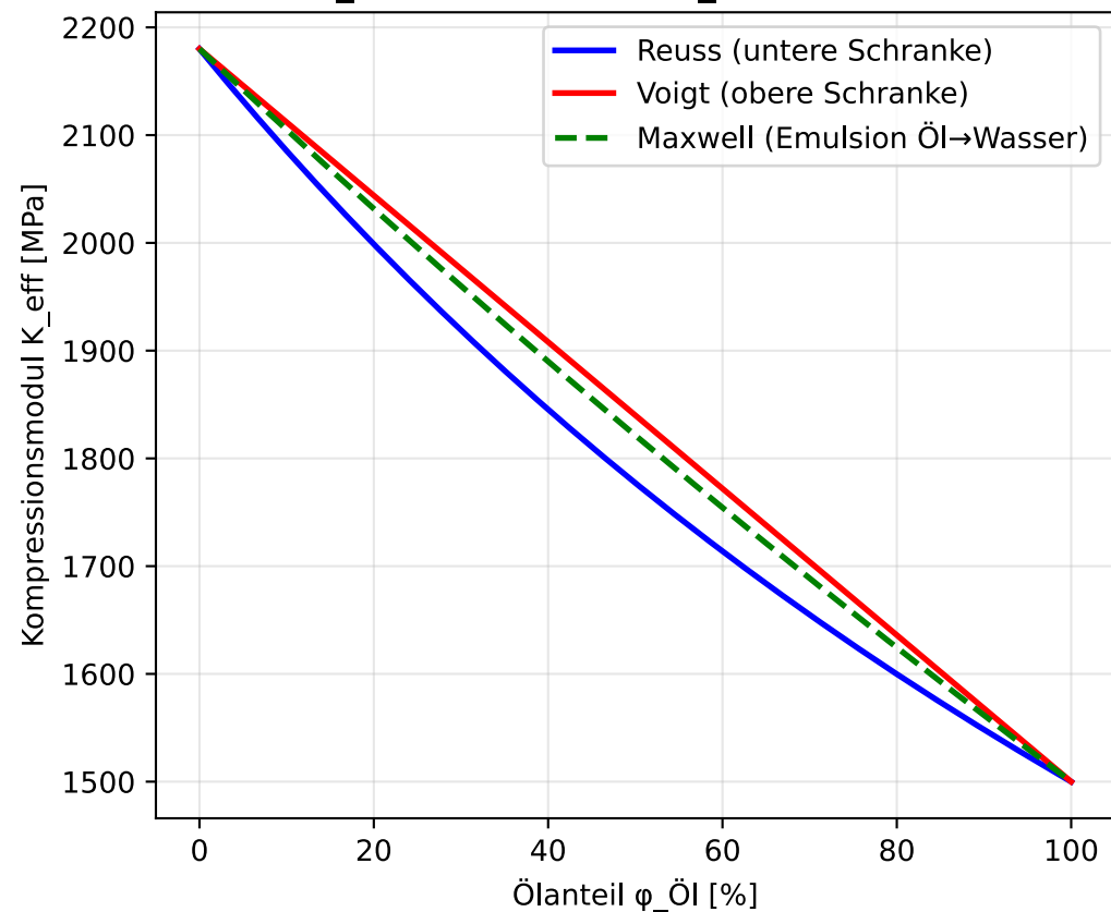
Experiment 10 – Mischungsregeln & Flüssigkeitsvergleich Mischungsregeln: Öl-Wasser-System ( K_{\text{water}}=2180 \text{ MPa} , K_{\text{oil}}=1500 \text{ MPa} )
