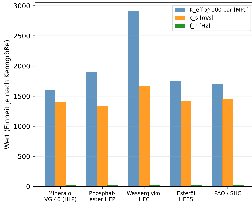
Flüssigkeitsvergleich: K , c_s , f_h ( A=20 \text{ cm}^2 , m=200 \text{ kg} , \bar{V}=2 \text{ l} )
