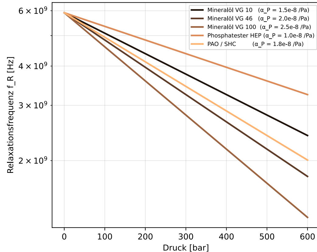
Abnahme der Relaxationsfrequenz mit Druck
