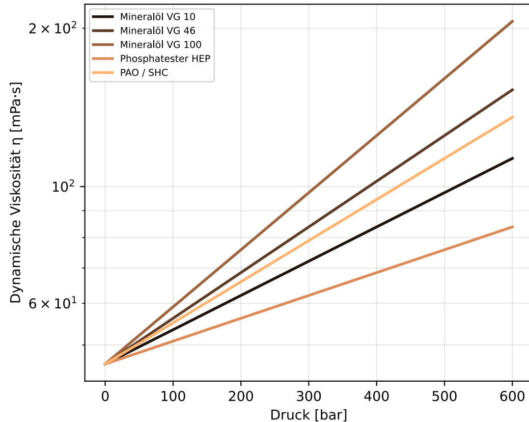
Barus: \eta(P) - exponentieller Anstieg
