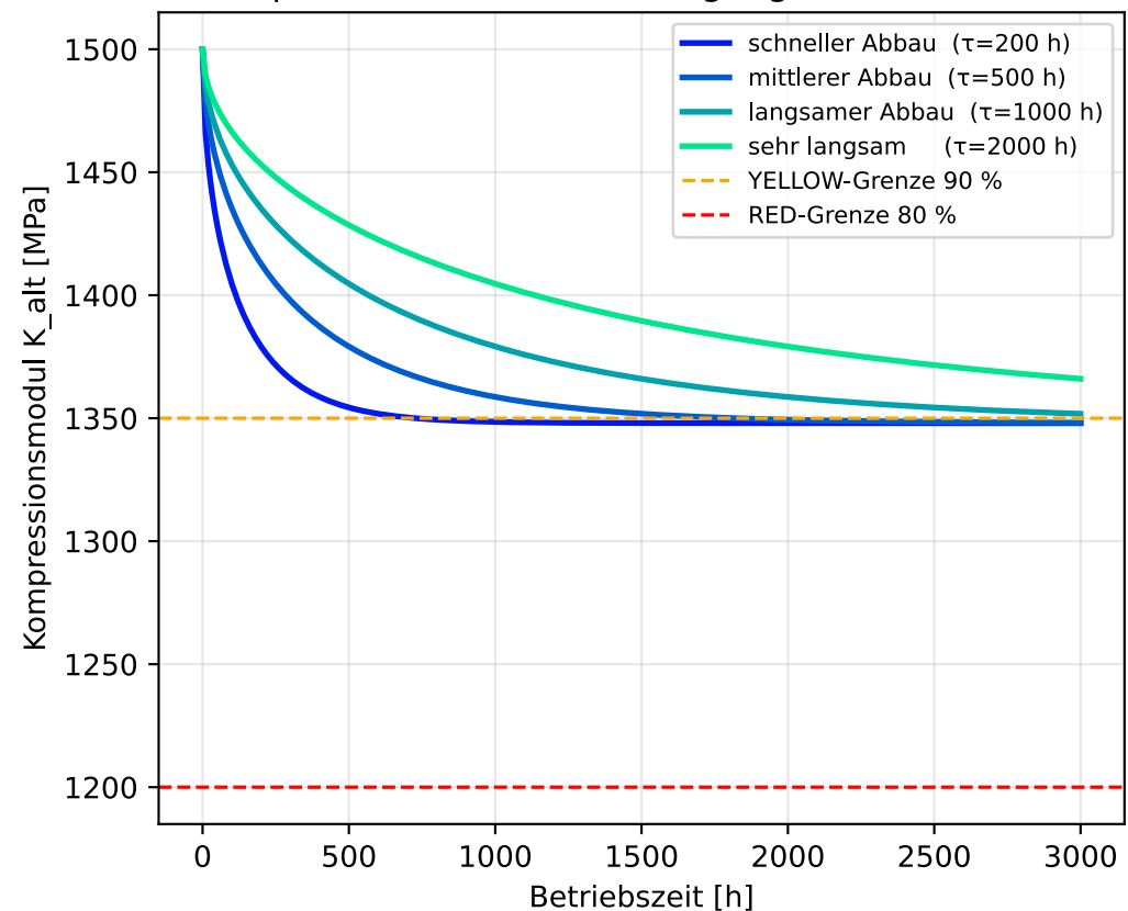
Korrespondierender Modulrückgang durch Scherabbau
