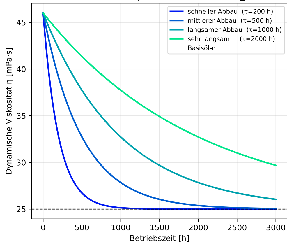
VII-Scherabbau: \eta(t) für verschiedene \tau_{\text{Sch}}
