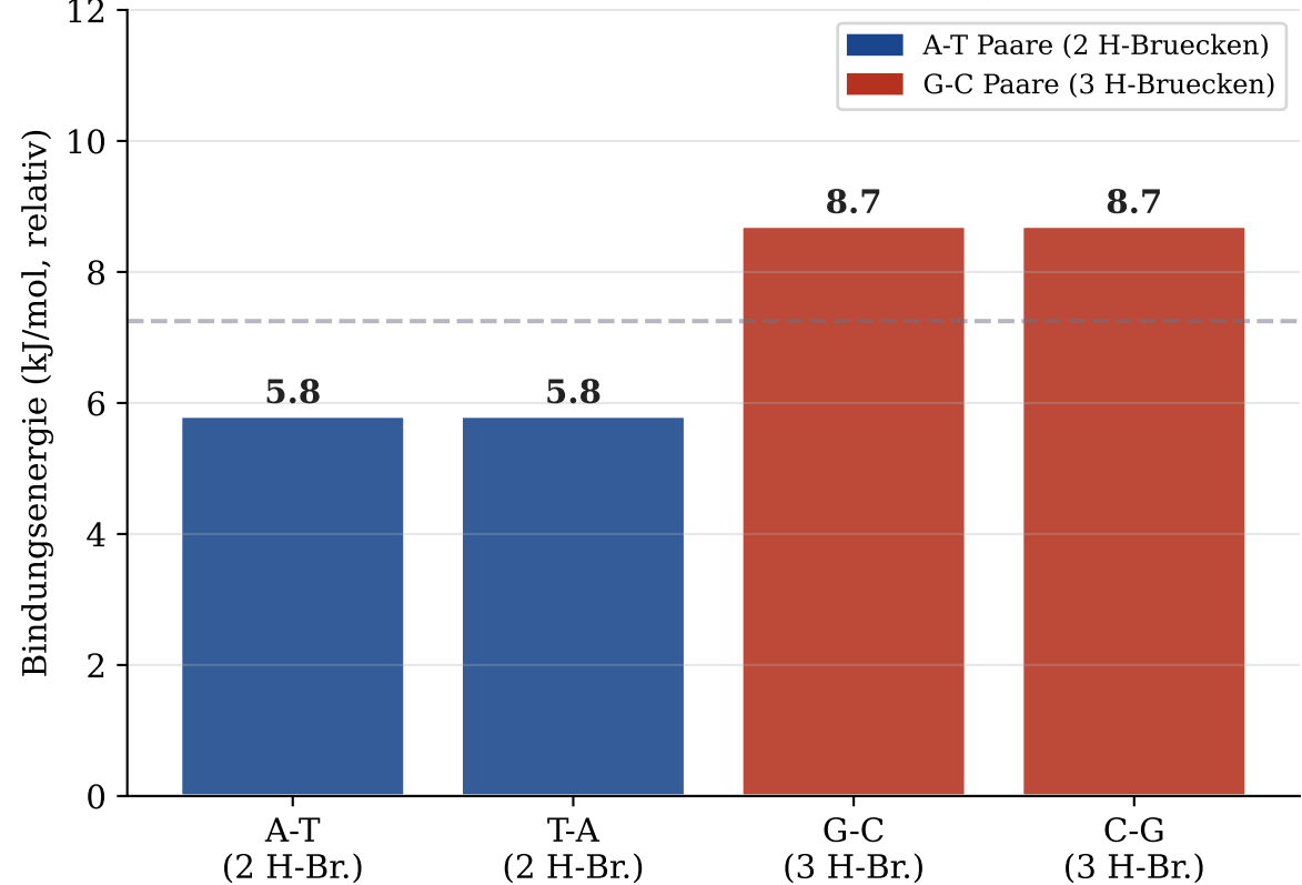
(a) Watson-Crick-Basenpaar-Bindungsstaerke
