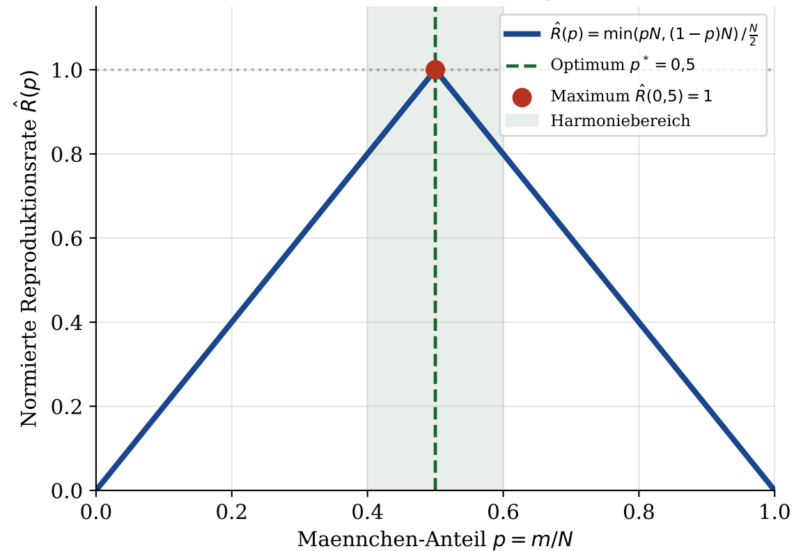
(a) Reproduktionsoptimum bei Paarungsharmonie ( p^* = 0,5 )
