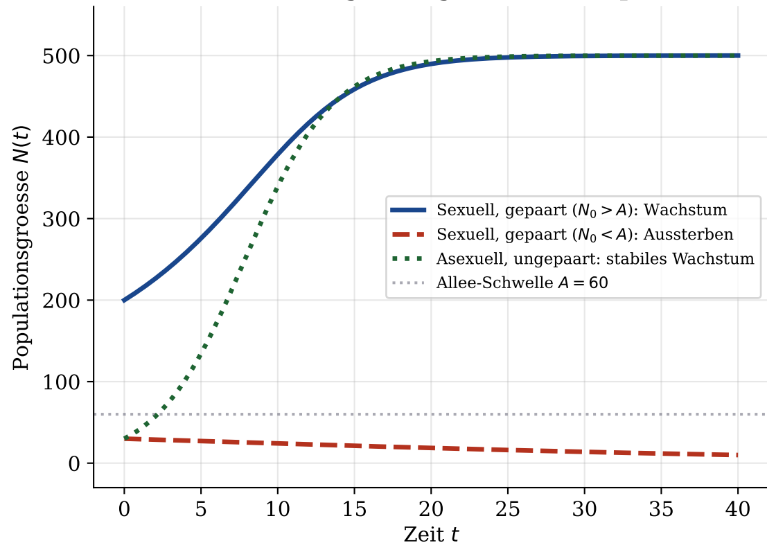
(b) Allee-Effekt: Paarung bedingt kritische Populationsdichte
