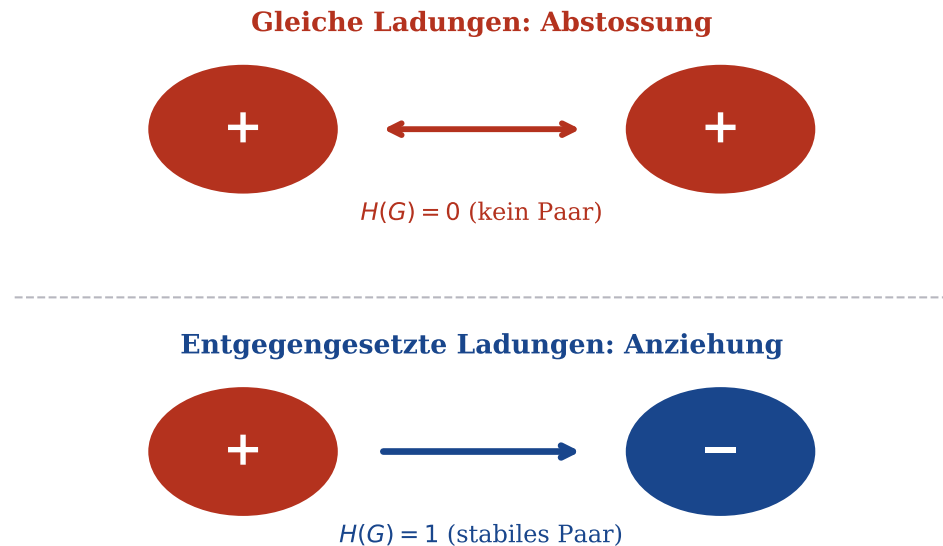
(b) Ladungspaare: Harmonie vs. Disharmonie
