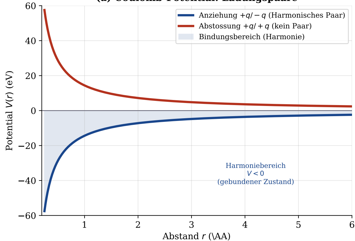
(a) Coulomb-Potential: Ladungspaare
